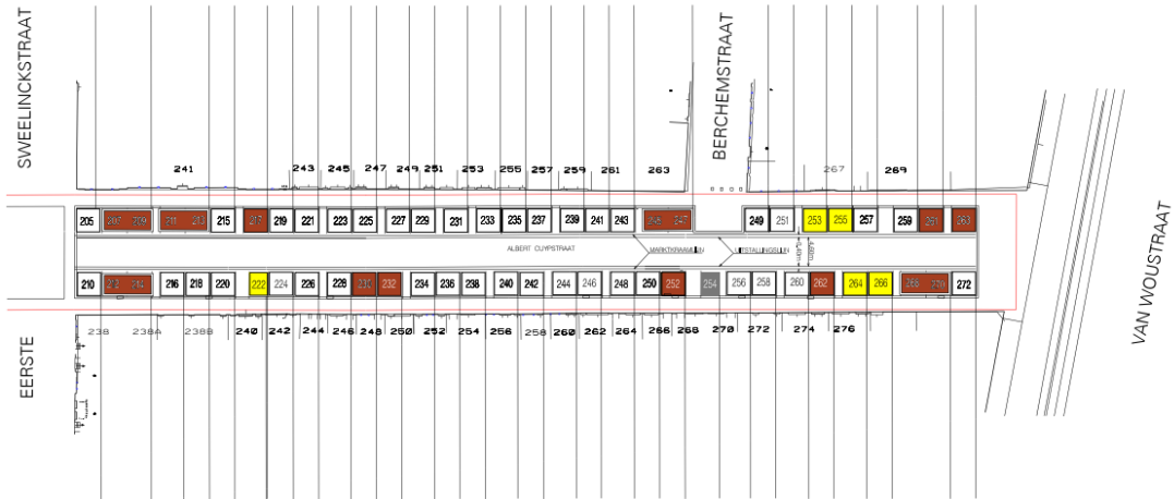
Inrichtingstekening als bijlage bij het Inrichtingsbesluit Albert Cuypmarkt, d.d. 19 12 2017
