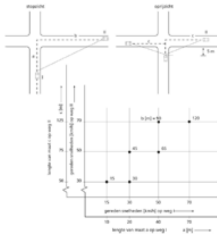
Figuur 10.1/11. Uitzichtdriehoeken
