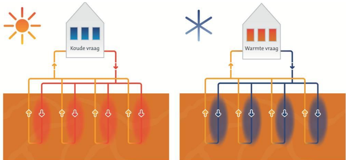
Afbeelding 2. Gesloten bodemenergiesysteem
