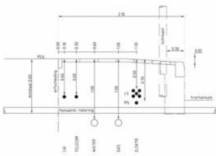
Standaarddwarsprofiel Bebouwde kom:
