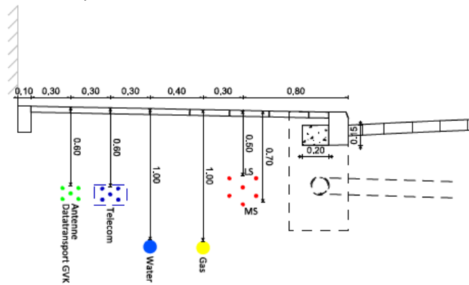
Standaarddwarsprofiel Bebouwde kom:
