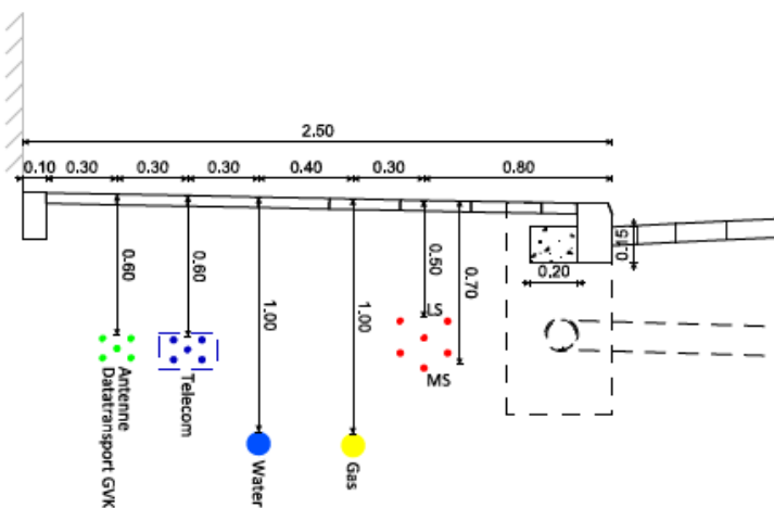
Standaarddwarsprofiel Industrie:
