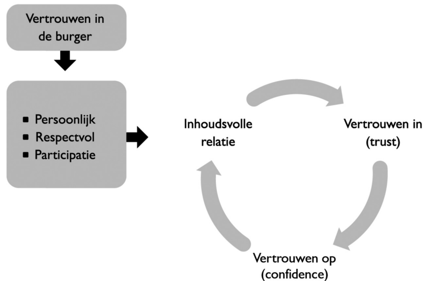
Figuur 3 Vertrouwensmodel
