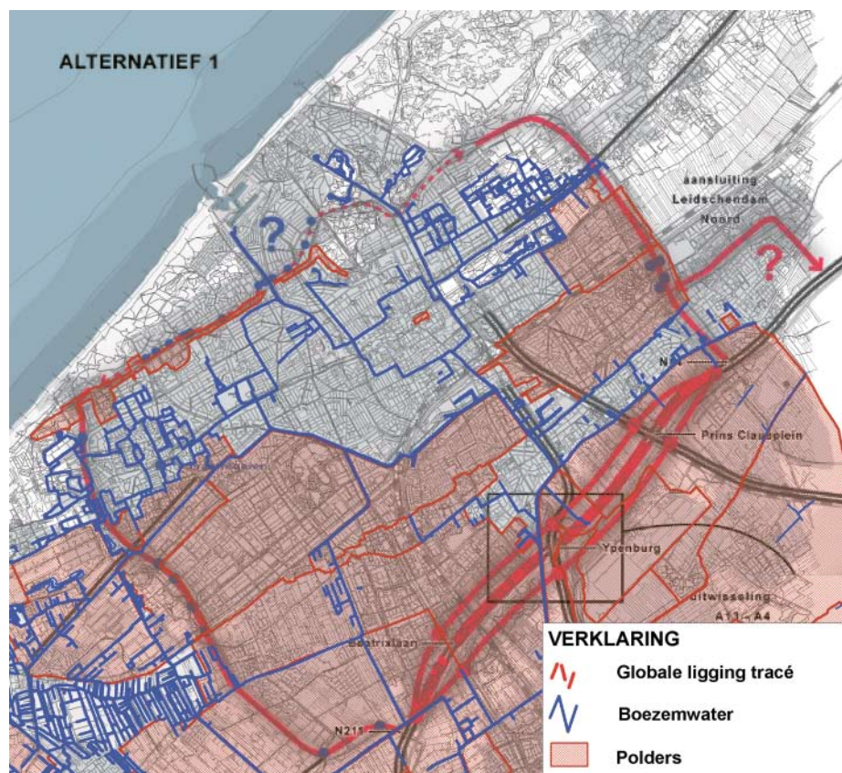
Figuur 18 Oppervlaktewatersysteem
