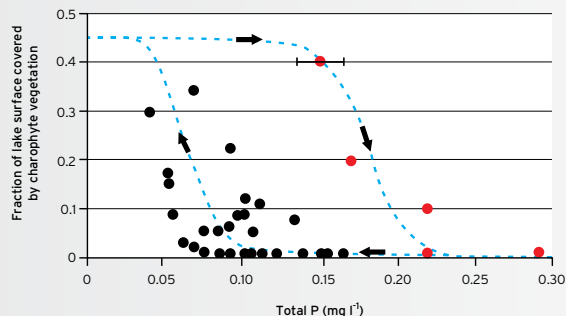
▲ Figuur 8: Reactie van de kranswervegetatie in het Veluwemeer op toe- en vervolgens een afname van de fosfaatconcentratie. De rode stippen laten zien dat de kranswieren zich bij een toenemende concentratie rond 1970 nog lang konden handhaven, maar toen ook snel verdwenen. De zwarte stippen laten zien dat de kranswieren zich pas in de jaren 90 bij een veel lagere concentratie weer konden herstellen.
