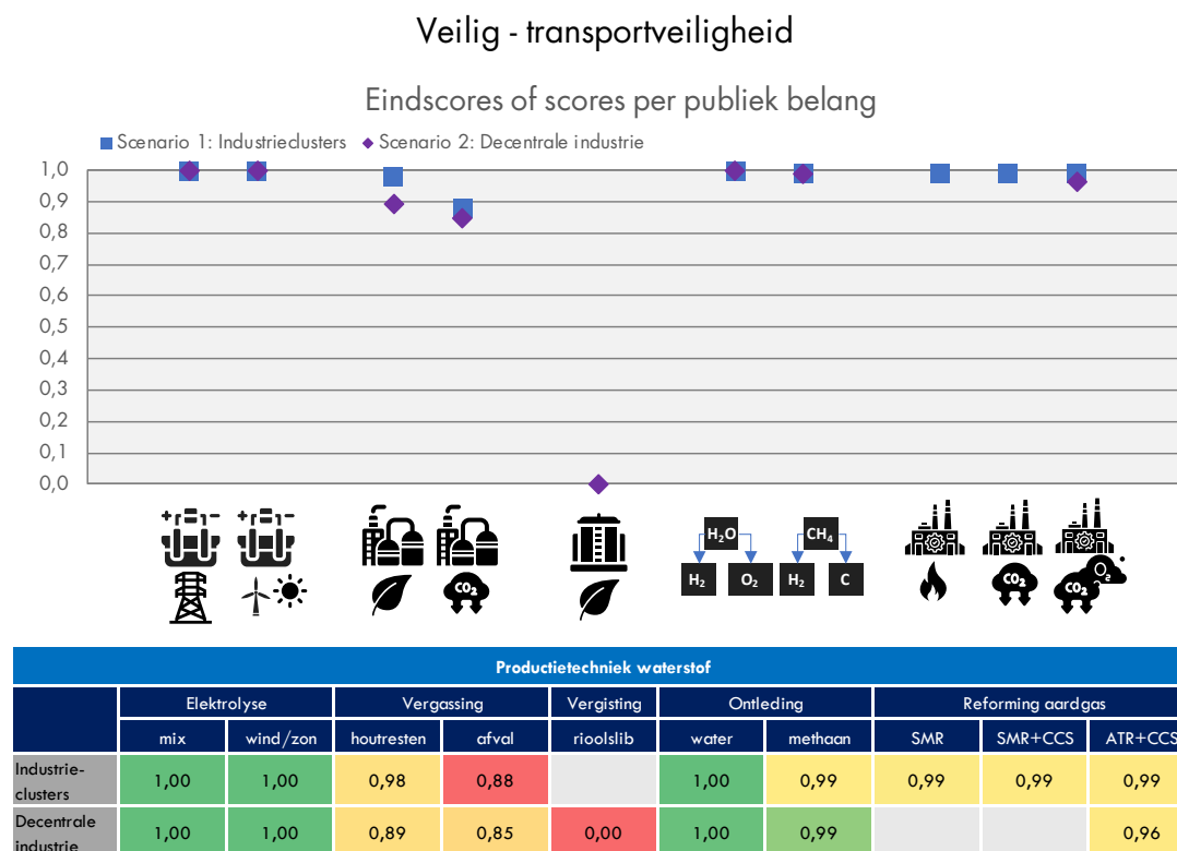
Figuur 12: Scores waterstofproductietechnieken op Transportveiligheid voor scenario 1 en 2
