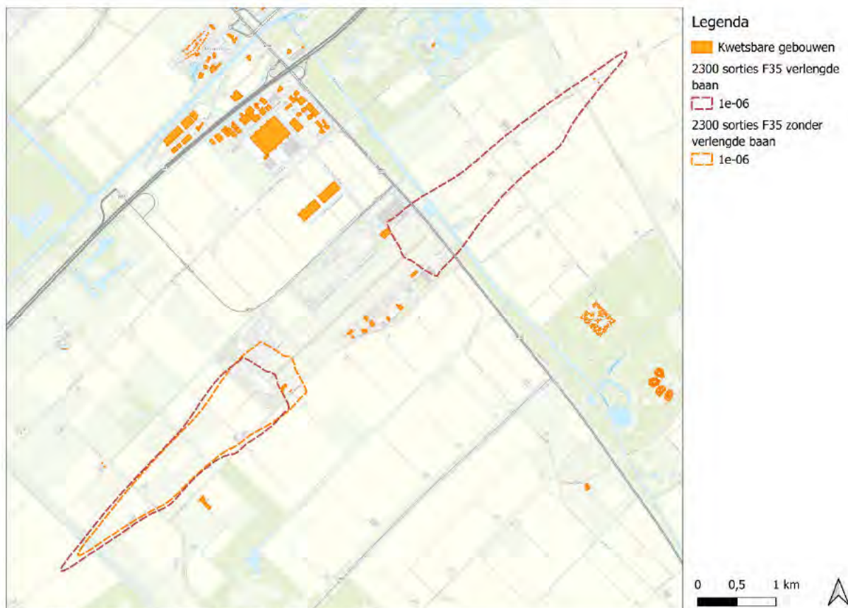
Figuur 2-6 PR10-6 contouren 2.300 sortjes F35 zonder en met verlengde baan
