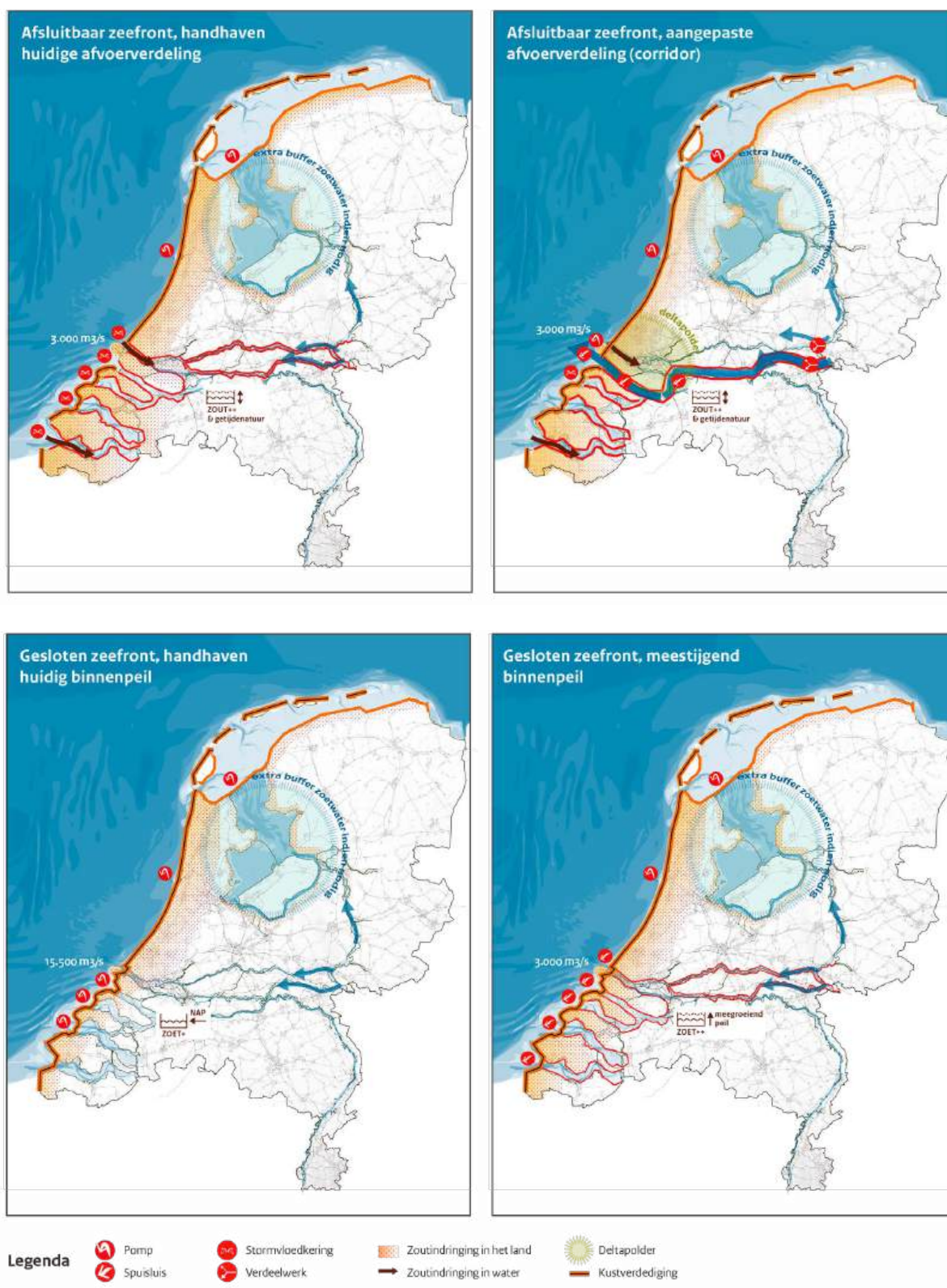
Figuur 4: De onderzochte 4 strategieën van de denkrichting Beschermen: afsluitbaar zeefront met stormvloedkeringen, meestijgend waterpeil en al dan niet aangepaste afvoerverdeling Rijntakken. En gesloten zeefront met hetzij pompen en een laag waterpeil, of spuien en een meestijgend waterpeil om overtollig rivierwater naar zee af te voeren. Door de verschillende combinaties van bouwstenen verschillen de strategieën in optredende verzilting en benodigde dijkversterkingen.
