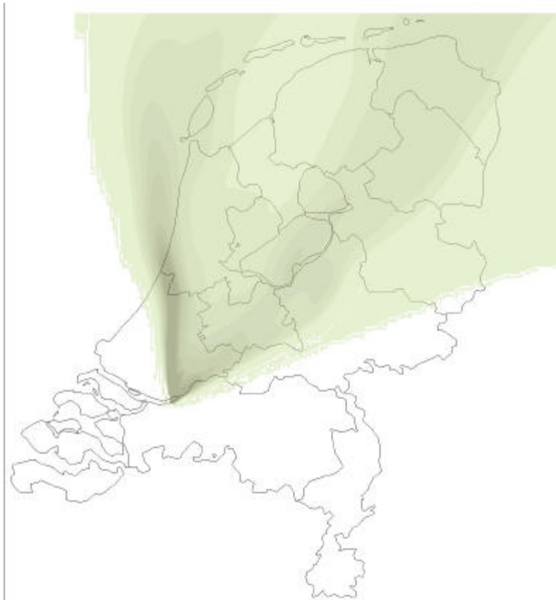
Figuur 2 Relatieve, over de brandperiode gesommeerde luchtconcentraties op leefniveau (relatieve eenheden)
