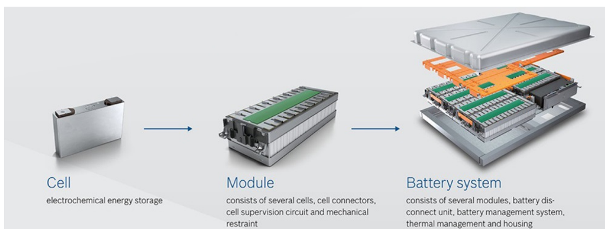
Figuur 1 Samenstelling batterijsysteem Bron: https://www.fic.com.tw/battery-management-system_p8.html
