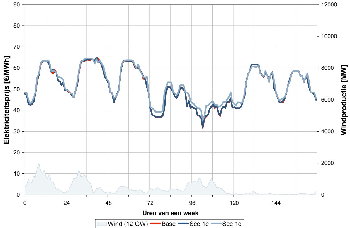
Figuur 8 Prijzen en windproductie voor een periode met weinig wind, vergelijking tussen scenario's met 12, 9 en 6 GW windcapaciteit. Het windvermogen is aangegeven als blauw vlak en de lijnen geven de prijzen in de verschillende scenario's.
