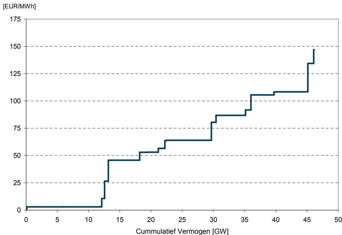
Figuur 2 Aanbod curve van het productiepark in Nederland in 2020 (brandstofmix volgens ENTSO-E SAF 2008)
