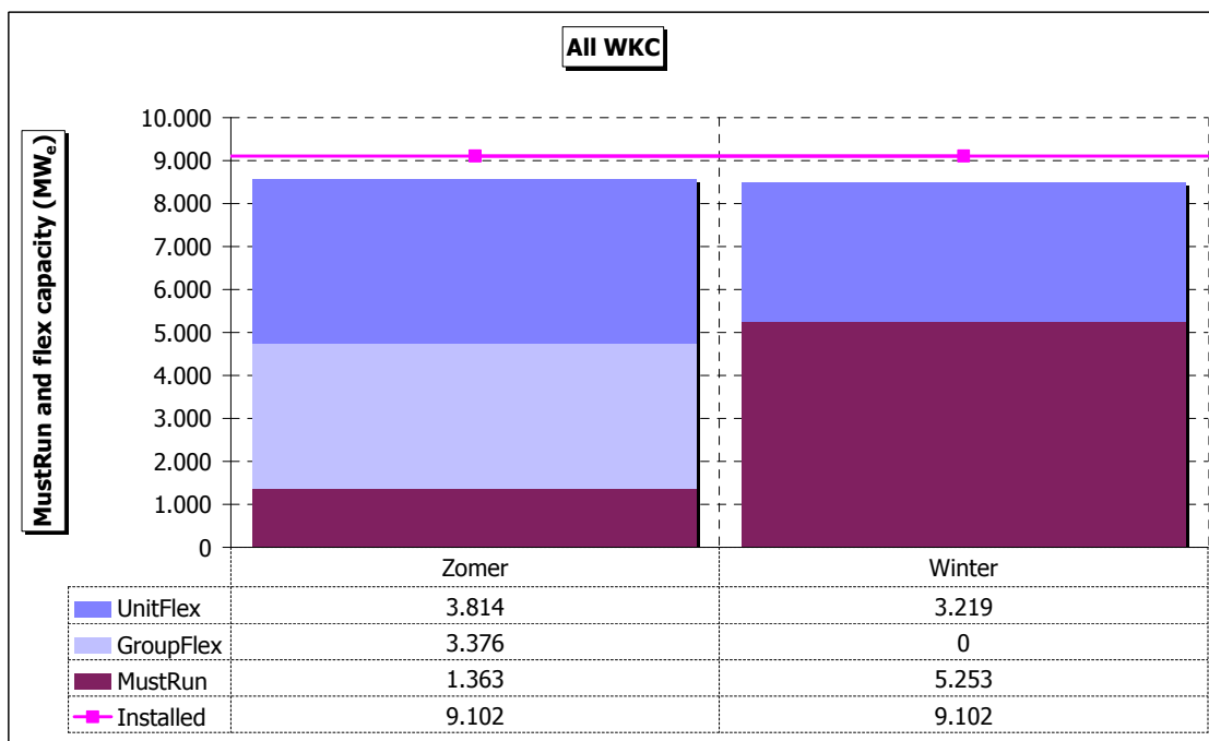
Figuur 23 Flexibiliteit van gezamenlijke WKC eenheden (GM NIET volledig flexibel), met de flexibiliteit van alle eenheden tezamen, zonder eenheden af te schakelen (Unitflex), de flexibiliteit waarbij eenheden worden afgeschakeld (Groupflex), en de minimale must run van alle gezamenlijke WKC eenheden.
