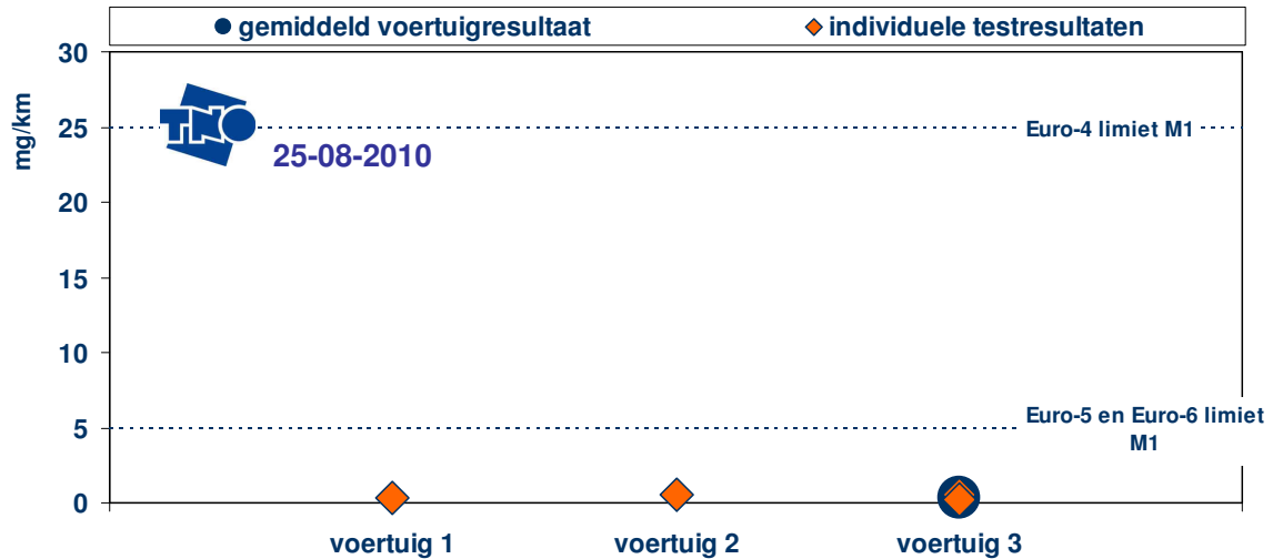
Figuur 6: fijn stof-emissie (PM) tijdens de typekeurtest
