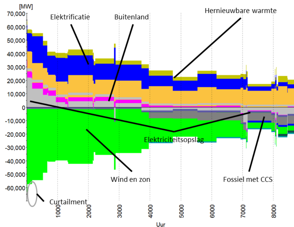
Figuur 2.11. elektriciteitsbalans bij variërend aanbod intermitterent hernieuwbaar, 80% reductie standaardvariant.
