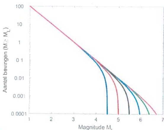
Figuur 3. Illustratie van een getrunkeerde M_{max} verdeling in de frequentie magnitude grafiek, waarbij de lijnen van links naar rechts maximale magnitudes vertegenwoordigen van 4,5; 5,0; 5,5; 6,0; 6,5 en 7,0..
