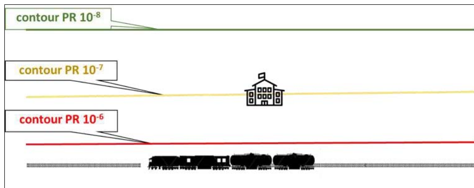
Figuur 2.2 Groepsrisico:
