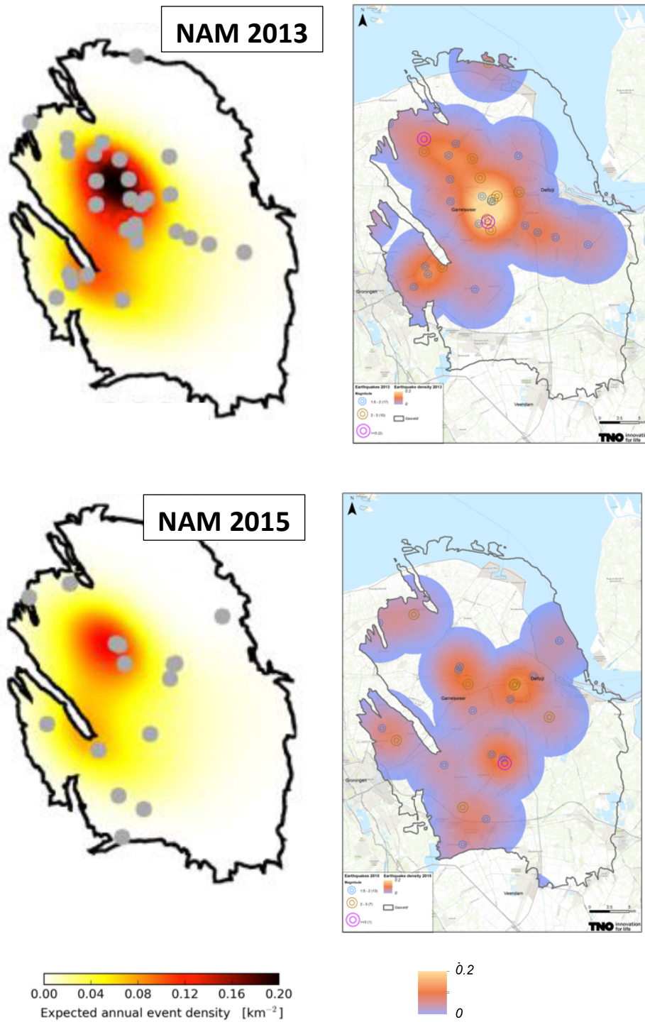
Figuur III-0-3: Aardbevingdichtheidskaarten ( M \geq 1,5 ) voor 2013 (boven) en 2015 (onder). Links is de modelvoorspelling van NAM gegeven, rechts de waarnemingen zoals in kaart gebracht door TNO.
