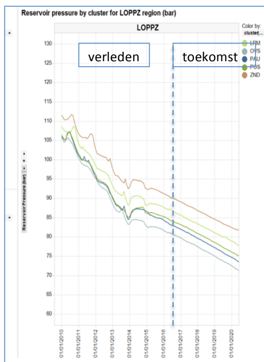
Figuur 7-1: Drukontwikkeling Loppersumgebied sinds 2010. Na de ingreep in januari 2014 is de druksdaling langzamer en gelijkmatiger. Bron: NAM
