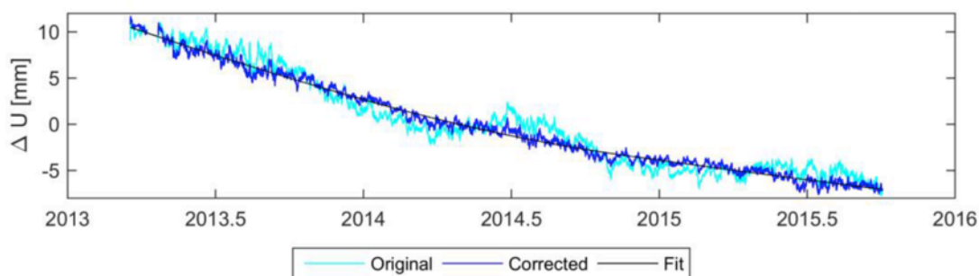
Figuur 6-1: De dalingsnelheid bij Ten Post, in het centrumgebied neemt met ongeveer een factor 2 af na de productie ingreep van januari 2014. Bron: TUDelft
