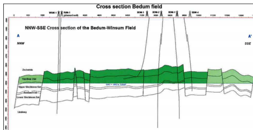
Figuur J.2 Doorsnede van het Bedum gasveld (Winningsplan Bedum, NAM 2010).
