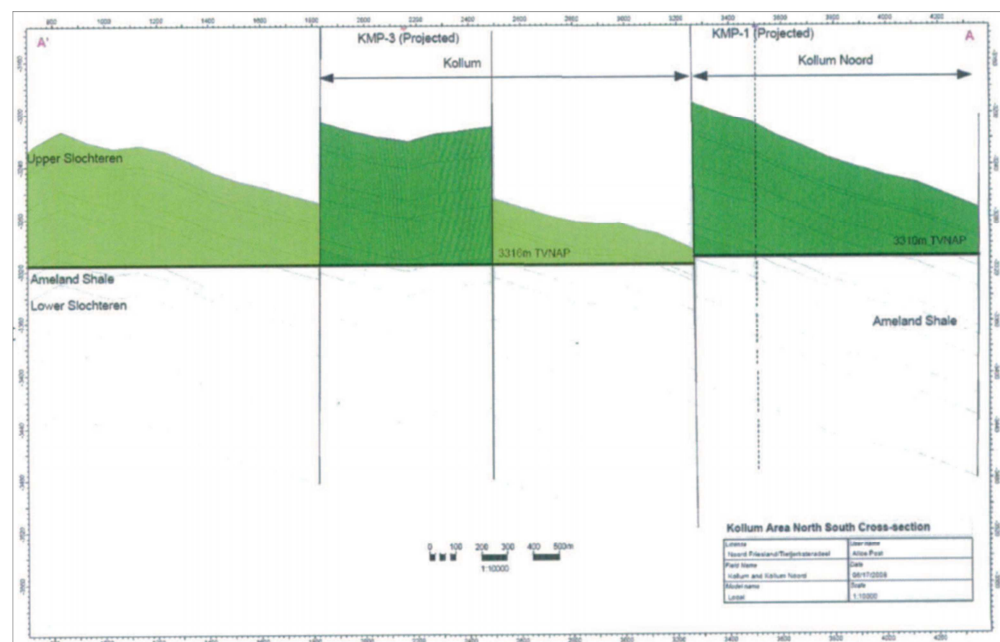
Figuur KK.2 Doorsnede van het Kollum en Kollum-Noord veld (Winningsplan Kollum, NAM 2012).
