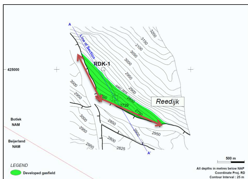
Figuur JJJ.1 Structuurkaart van het Reedijk gasveld ( www.nlog.nl ). De diepte contourlijnen representeren de bovenkant van de Hoofd-Bontzandsteen Subgroep.
