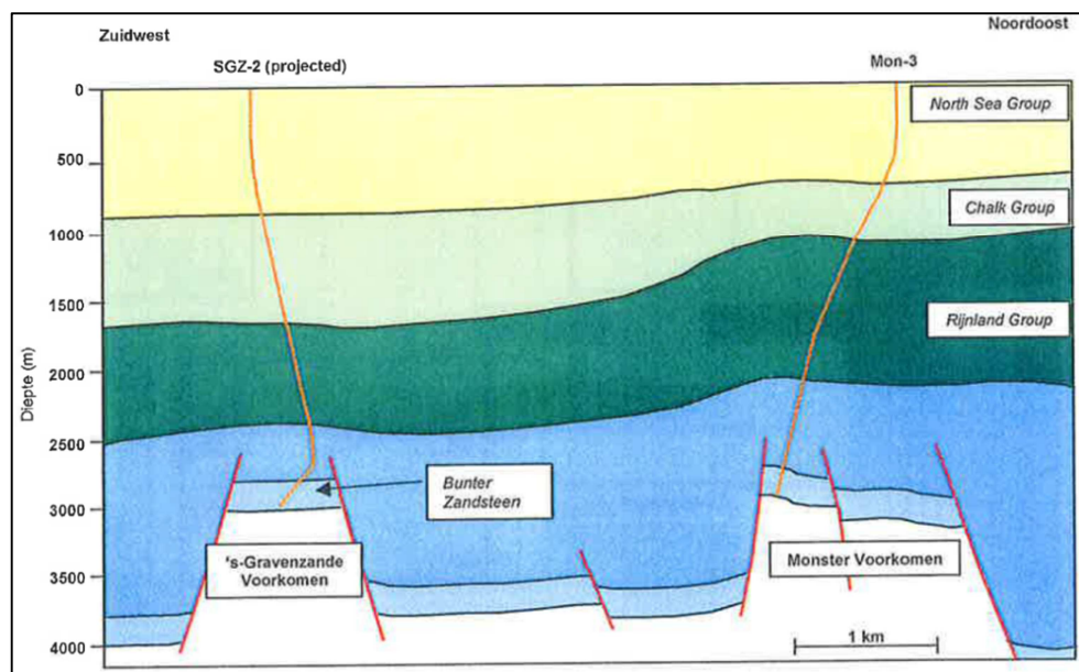
Figuur LLL.2 Doorsnede van het 's-Gravenzande gasveld (Winningsplan Gaag-Monster, NAM 2013).
