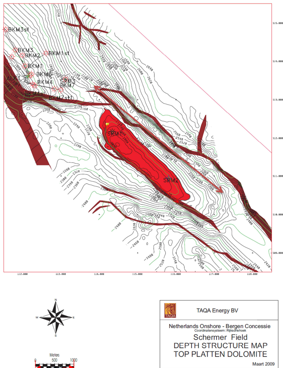
Figuur 000.1 Structuurkaart van het Schermer gasveld ( www.nlog.nl ).
