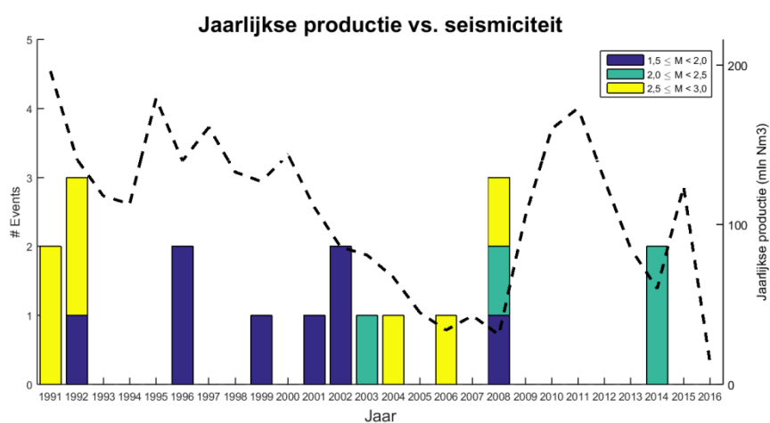
Figuur W.3 Geïnduceerde seismiciteit ( M_L \geq 1,5 ) vanaf 1991 voor het Eleveld gasveld in de tijd gerangschikt naar magnitude alsook de jaarlijkse productie (miljoen Nm³).
