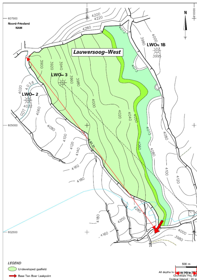
Figuur MM.2 Structuurkaart van het Lauwersoog West voorkomen ( www.nlog.nl ). De diepte contourlijnen representeren de bovenkant van het Boven-Slochteren laagpakket. (De lengte van de breuk is gegeven in inch en is later omgerekend naar kilometers).
