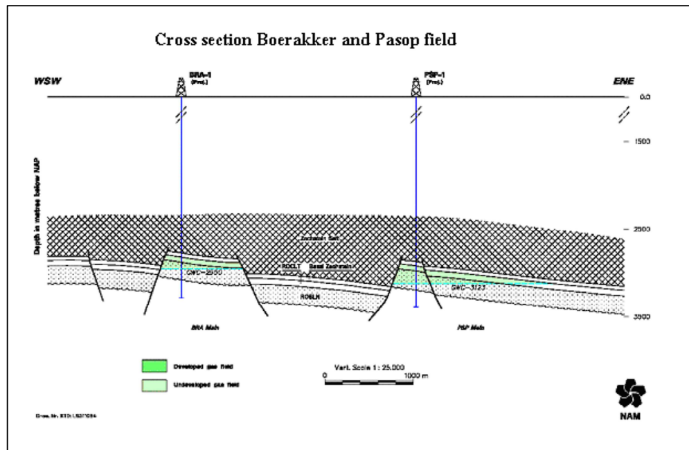
Figuur P.2 Doorsnede van de Boerakker en Pasop gasvelden (Winningsplan Grijskerk-Zuid, NAM 2005).
