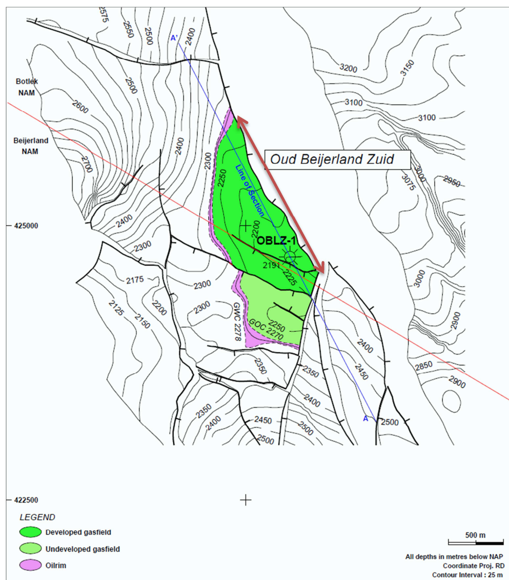
Figuur DDD.1 Structuurkaart van het Röt voorkomen van het Oud-Beijerland Zuid gasveld ( www.nlog.nl ). De diepte contourlijnen representeren de top van de Röt Formatie.
