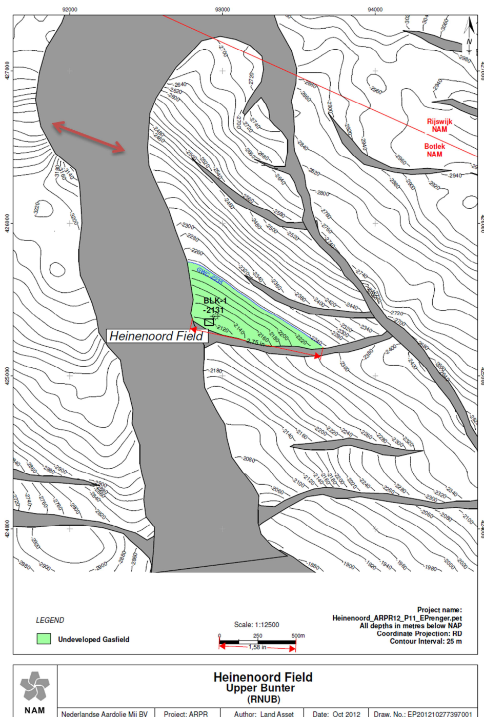
Figuur HH.1 Structuurkaart en doorsnede van het Heinenoord gasveld (Winningsplan Heinenoord, NAM 2013).
