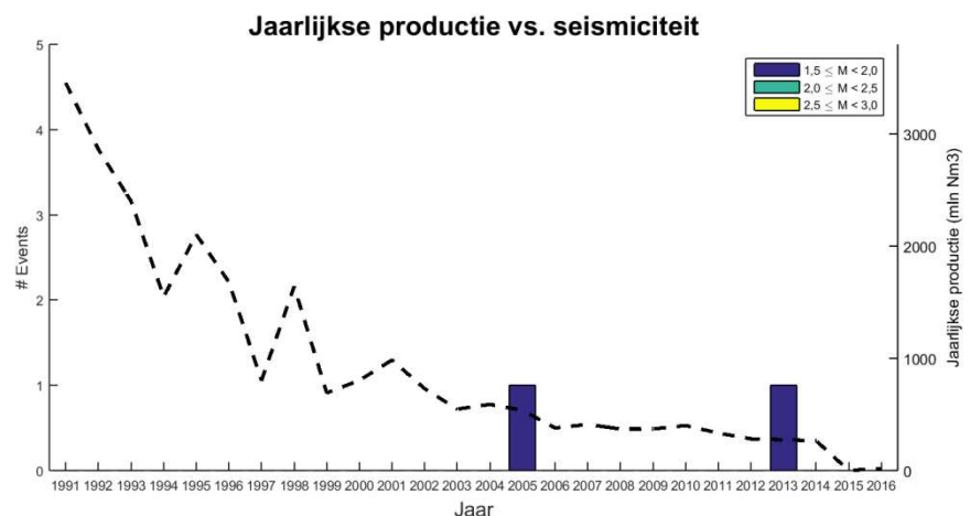
Figuur F.4 Geïnduceerde seismiciteit ( M_L \geq 1,5 ) voor het Ameland-Oost gasveld in de tijd gerangschikt naar magnitude alsook de jaarlijkse productie (mln. Nm 3 ).
