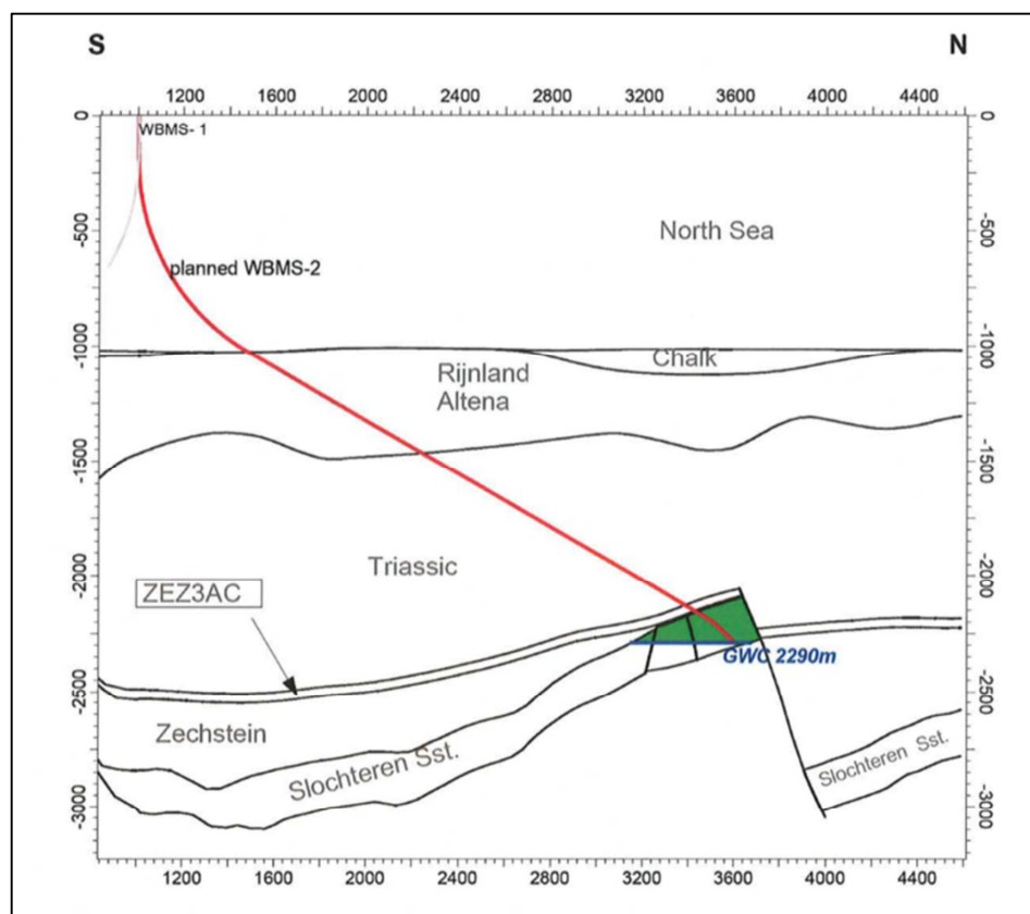
Figuur KKK.2 Doorsnede van het Rustenburg voorkomen (Winningplan Rustenburg, NAM 2009).
