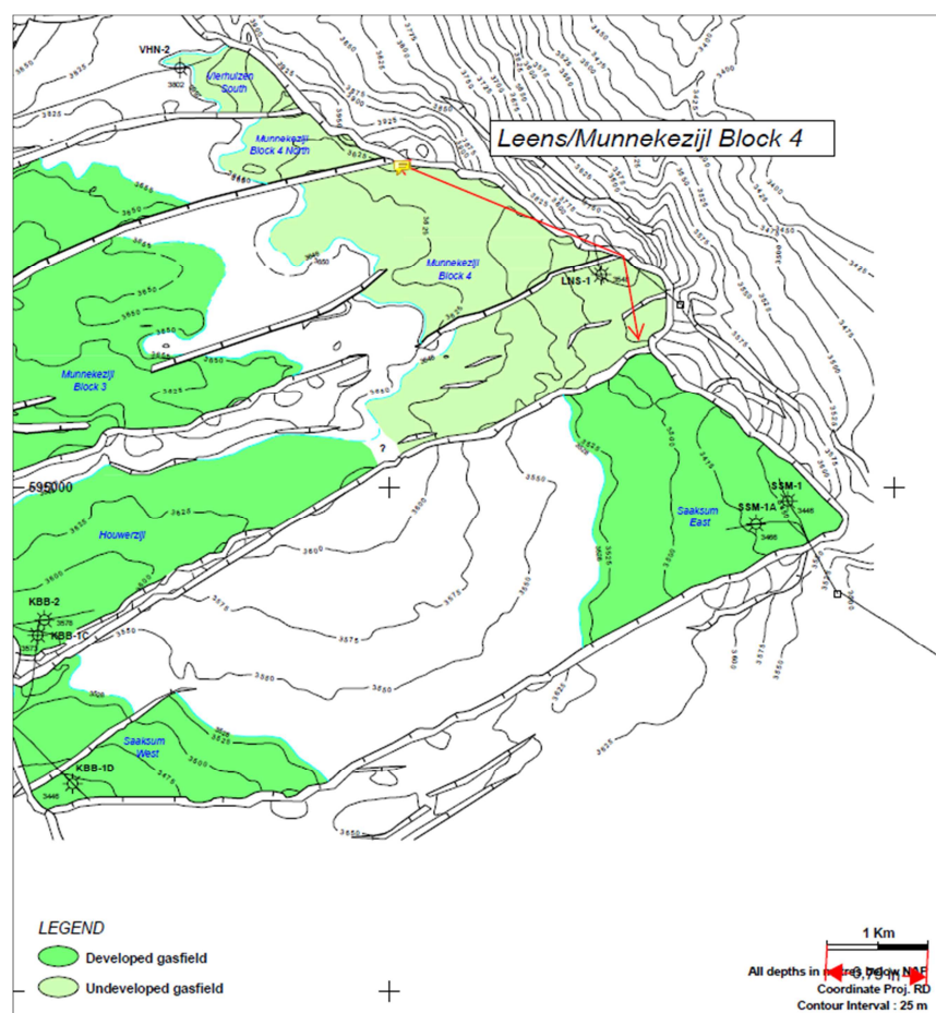
Figuur NN.1 Structuurkaart van het Leens gasveld ( www.nlog.nl ). De diepte contourlijnen representeren de bovenkant van het Boven-Slochteren Laagpakket. (De lengte van de breuk is gegeven in inch en is later omgerekend naar kilometers).
