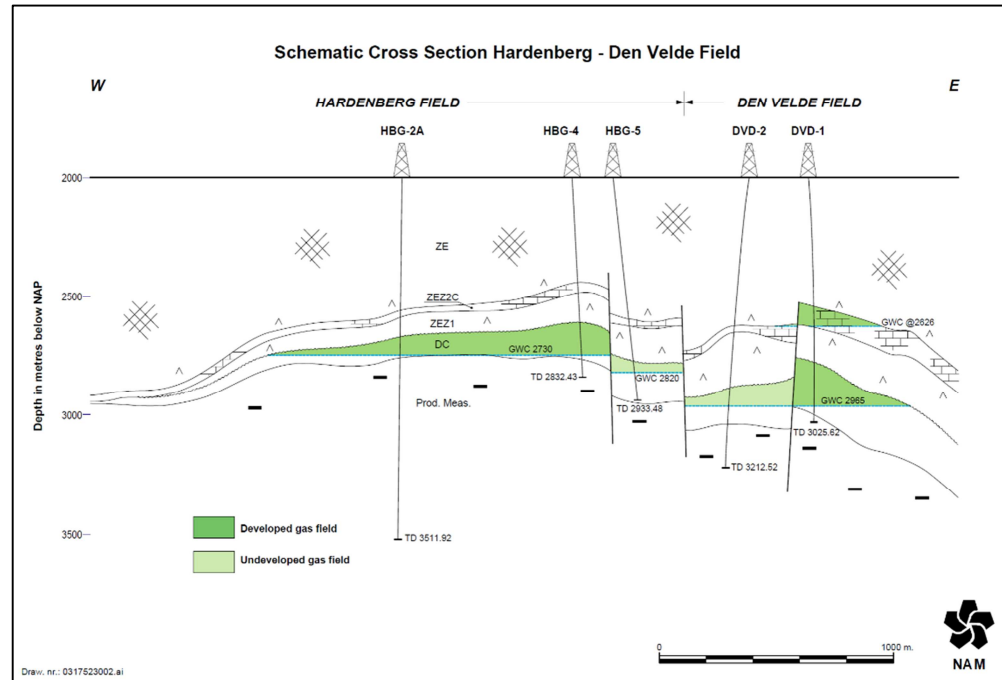
Figuur FF.2 Dwarsdoorsnede door het Hardenberg veld (Winningsplan Hardenberg, NAM 2012).
