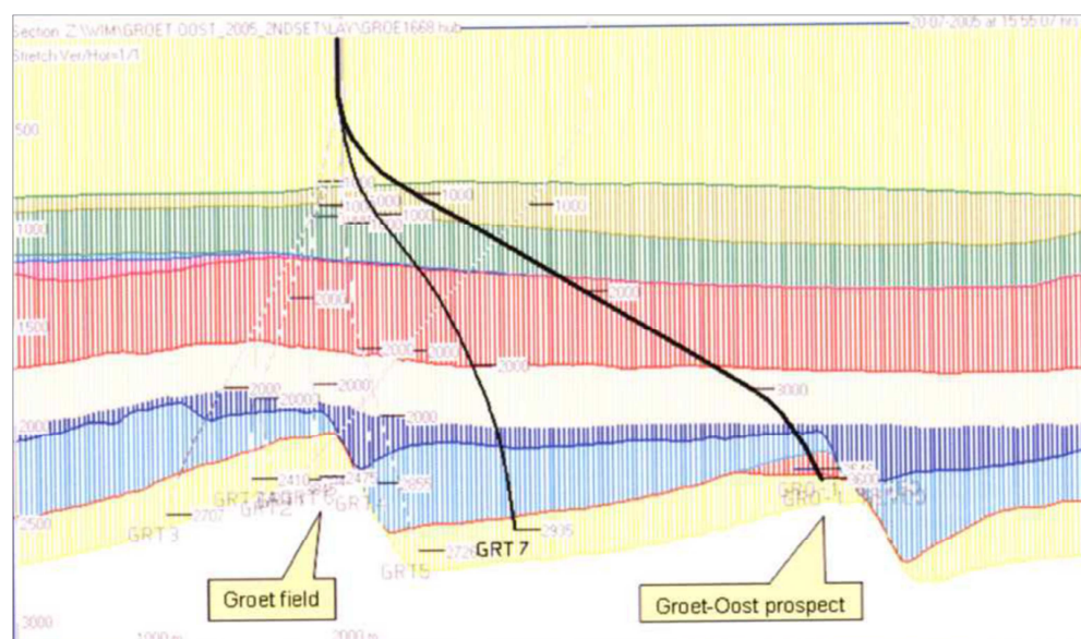
Figuur DD.2 Schematische doorsnede van het Groet en Groet-Oost veld waarin te zien is dat het hier om half graben structuren gaat (Winningsplan Groet-Oost, NAM 2005).
