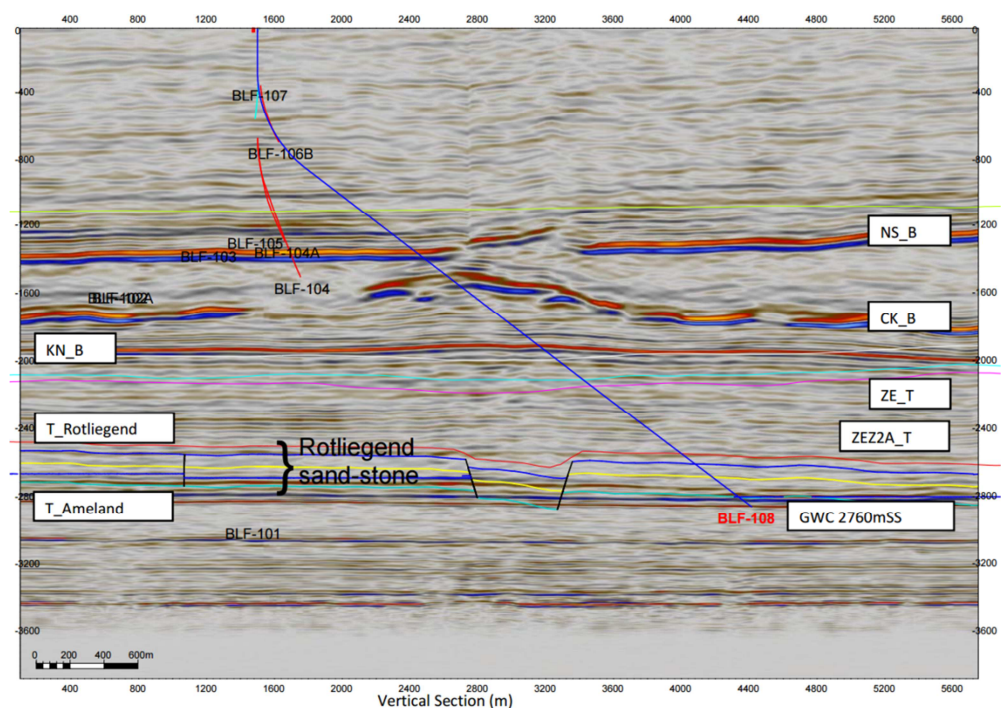
Figuur N.2 Seismische doorsnede van het Blija Zuidoost gasveld (Winningplan Blija-Zuid, NAM 2011). Het aangeduide GWC betreft een oude inschatting.
