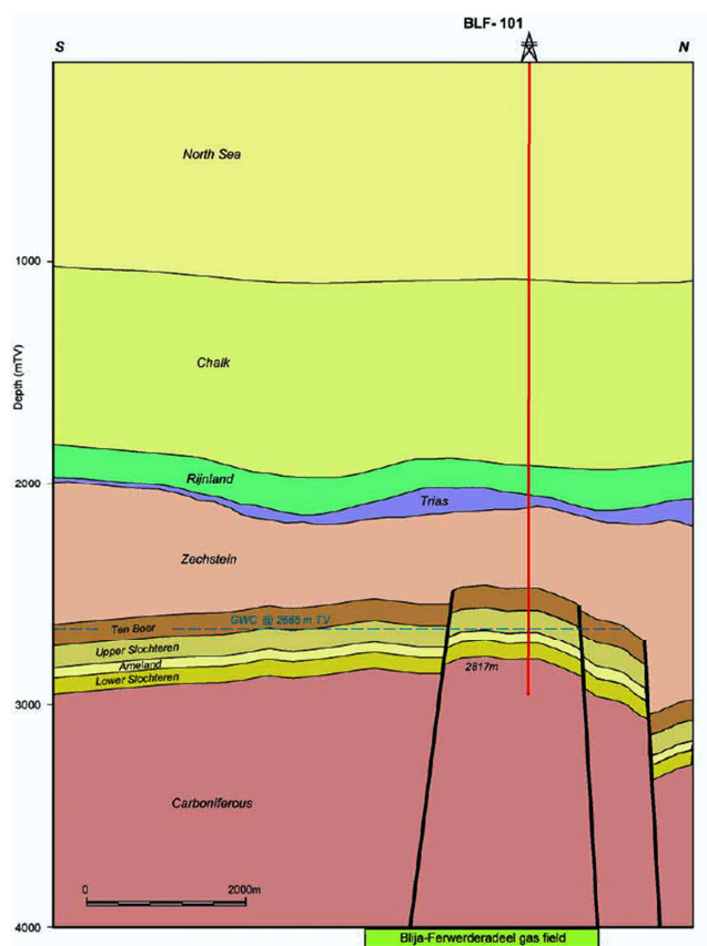
Figuur L.2 Doorsnede van het Blija-Ferwerderadeel gasveld (Winningsplan Blija, NAM 2003). De Boven-Rotliegend Formatie is onderverdeeld in meerdere eenheden.
