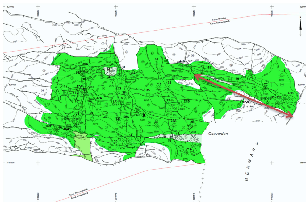
Figuur S.1 Structuurkaart van het ZE22C voorkomen van het Coevorden gasveld ( www.nlog.nl ). De diepte contourlijnen representeren de bovenkant van het ZE22C laagpakket.
