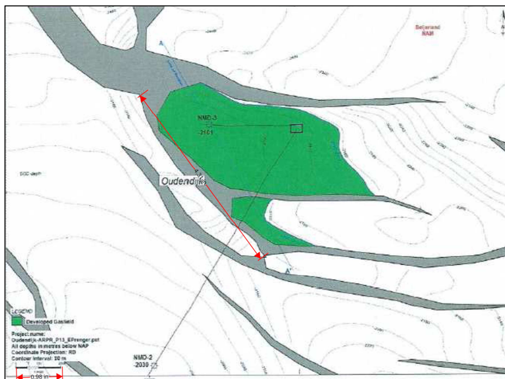
Figuur GGG.1 Structuurkaart van het Oudendijk gasveld (Winningplan Oudendijk, NAM 2014). De diepte contourlijnen representeren de bovenkant van de Röt Formatie. (De lengte van de breuk is gegeven in inch en is later omgerekend naar kilometers).
