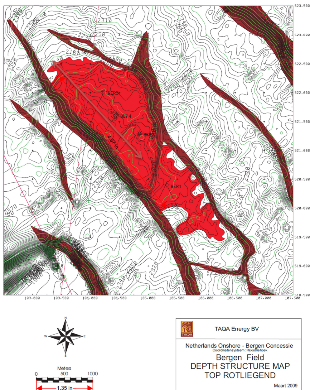
Figuur K.1 Structuurkaart van het Bergen gasveld ( www.nlog.nl ). De diepte contourlijnen representeren de bovenkant van het Boven-Slochteren Zandsteen Laagpakket.
