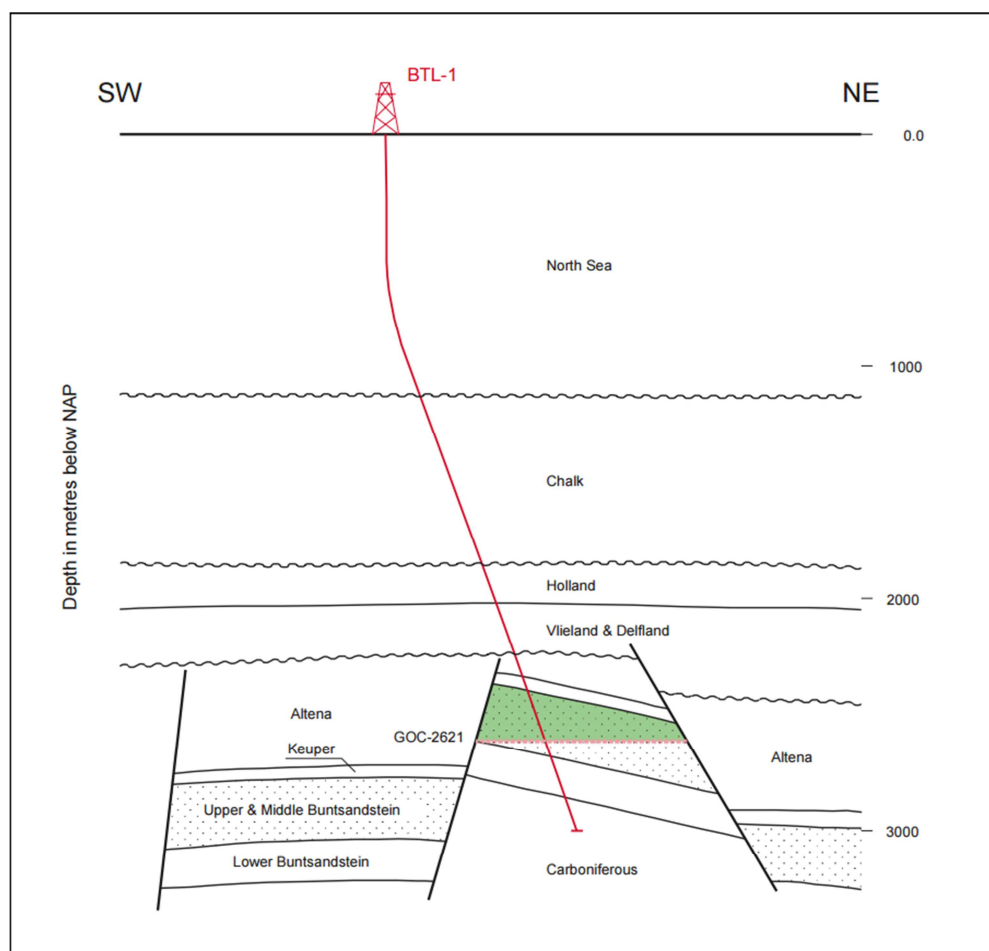
Figuur Q.2 Schematische doorsnede van het Botlek gasveld (Winningsplan Botlek, NAM 2003).
