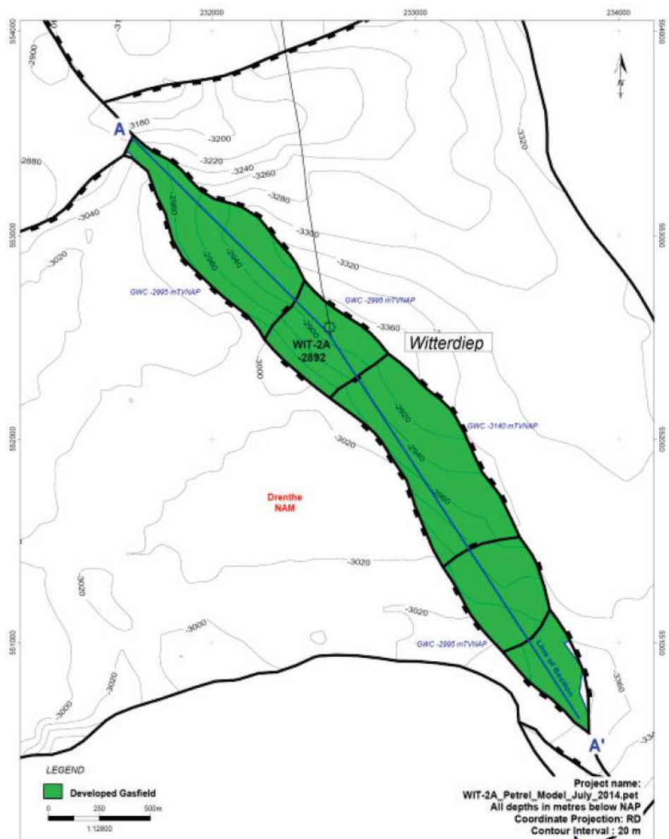
Figuur ZZZ.1 Overzichtskaart van het Witterdiep gasveld en omliggende velden (Winningsplan Westerveld, NAM 2016).
