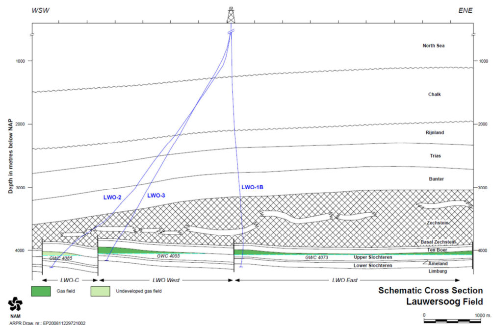
Figuur MM.3 Doorsnede van de Lauwersoog voorkomens (Winningsplan Lauwersoog, NAM 2011).
