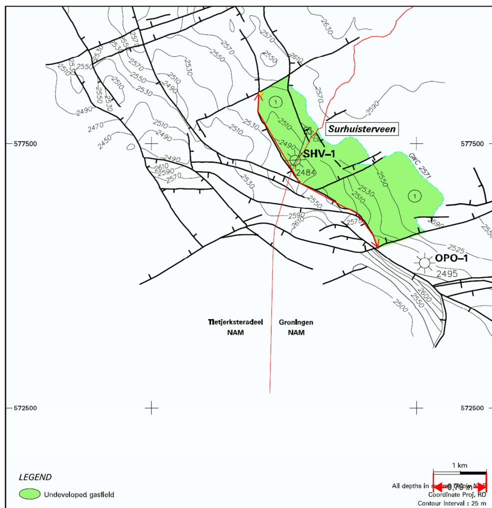
Figuur SSS.1 Structuurkaart van het Surhuisterveen gasveld ( www.nlog.nl ). De diepte contourlijnen representeren de bovenkant van het Boven-Slochteren Laagpakket. (De lengte van de breuk is gegeven in inch en is later omgerekend naar kilometers).
