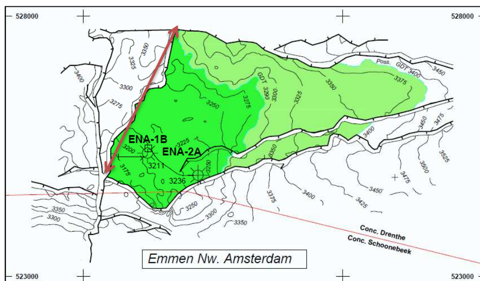
Figuur Y.1 Structuurkaart van het Emmen-Nieuw Amsterdam gasveld ( www.nlog.nl ). De diepte contourlijnen representeren de bovenkant van het ZE2C laagpakket.
