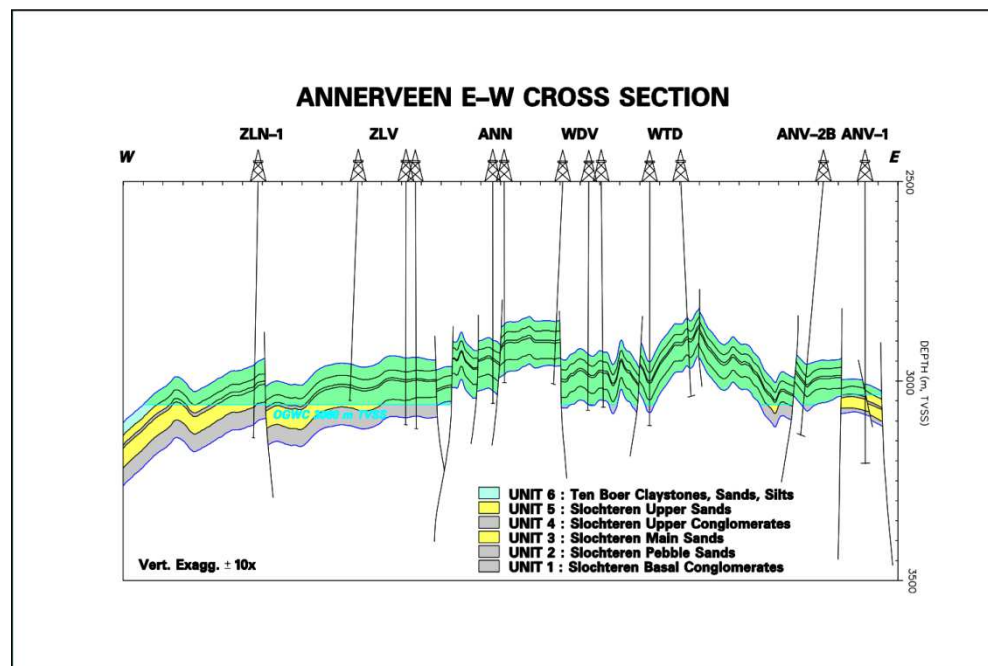
Figuur 1.2 Doorsnede van het Annerveen gasveld (Winningsplan Annerveen, NAM 2003).
