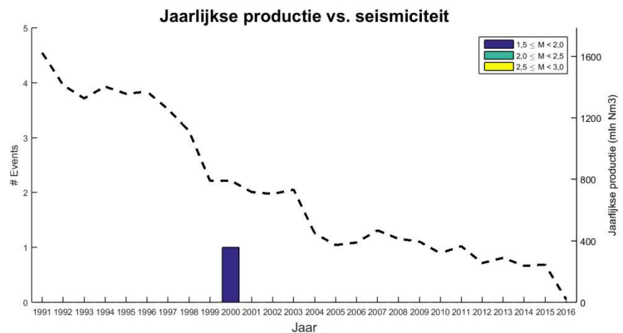
Figuur S.5 Geïnduceerde seismiciteit ( M_L \geq 1,5 ) voor het Coevorden gasveld in de tijd gerangschikt naar magnitude alsook de jaarlijkse productie (miljoen \text{Nm}^3 ).
