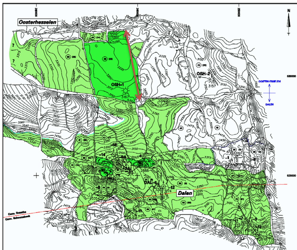
Figuur AAA.2 Structuurkaart van het DC voorkomen van het Oosterhesselen veld ( www.nlog.nl ). De scheiding tussen het Dalen en Oosterhesselen veld wordt gevormd door een grote oost-west georiënteerde breuk.
