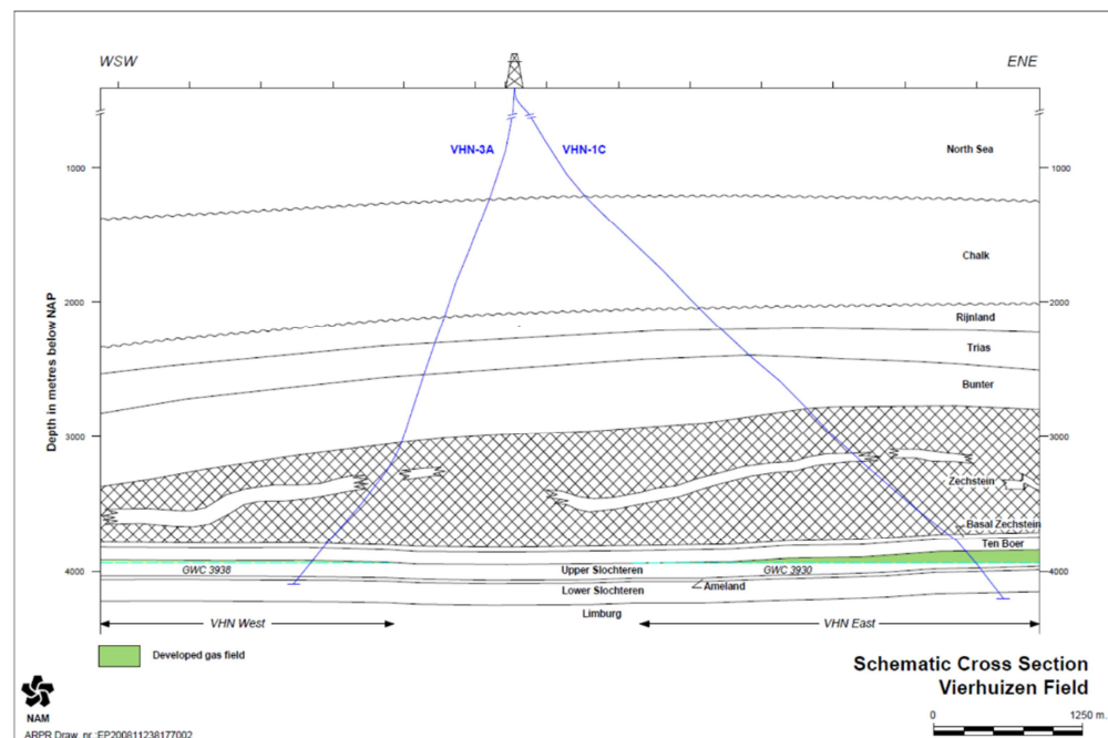
Figuur VVV.2 Doorsnede van het Vierhuizen veld (Winningplan Waddenzee, NAM 2011).
