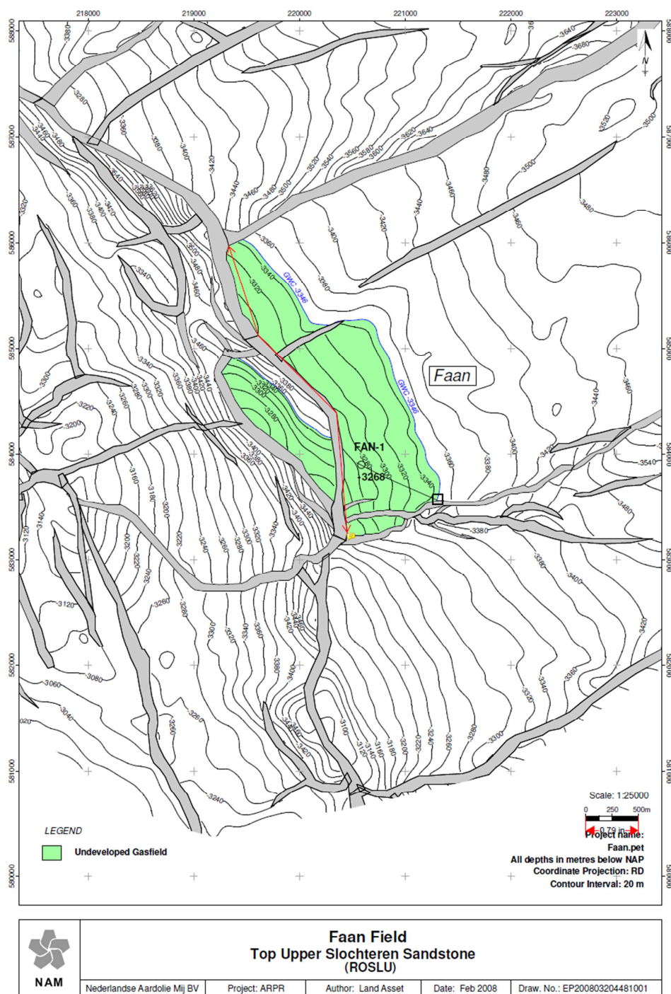
Figuur Z.1 Locatiekaart van het Faan gasveld (Winningplan Faan, NAM 2008). De diepte contourlijnen representeren de bovenkant van de Slochteren Formatie.
