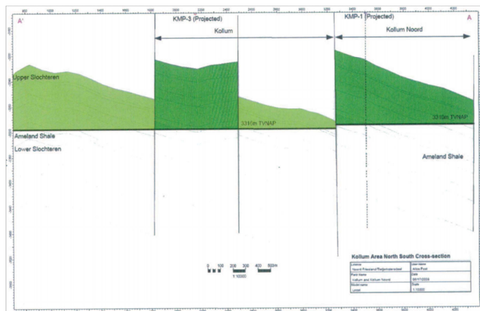
Figuur JJ.2 Doorsnede van het Kollum en Kollum-Noord veld (Winningplan Kollum, NAM 2012).
