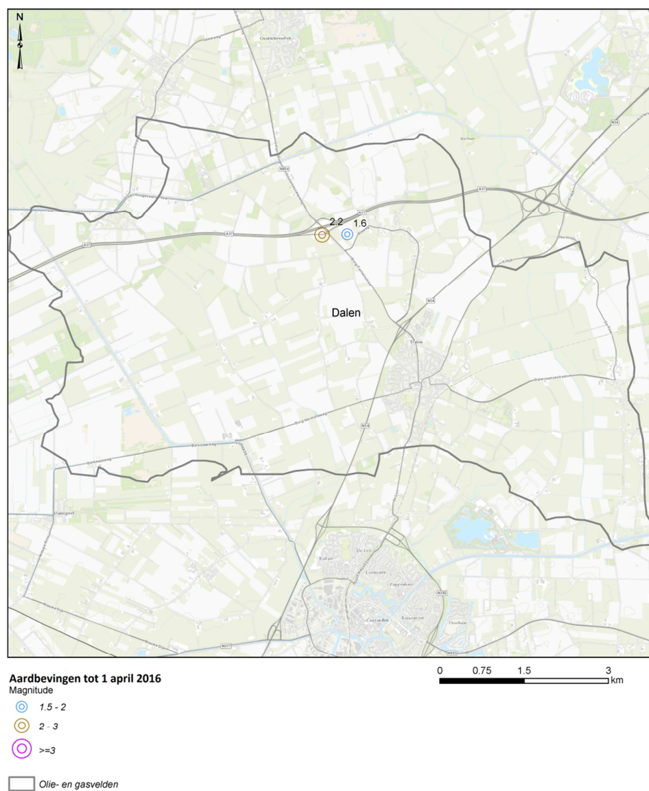
Figuur U.6 Geïnduceerde seismiciteit ( M_L \geq 1,5 ) voor het Dalen gasveld (zwarte contour).
