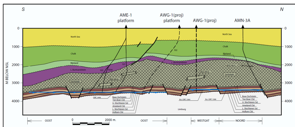
Figuur G.2 Doorsnede van de Ameland-Oost, -Westgat en -Noord gasvelden (Winningsplan Ameland, NAM 2011).
