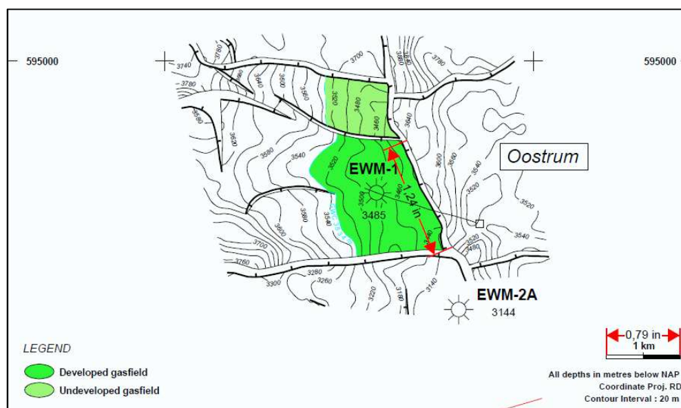
Figuur BBB.1 Structuurkaart van het Oostrum gasveld ( www.nlog.nl ). De diepte contourlijnen representeren de bovenkant van de Slochteren Zandsteen Formatie. (De lengte van de breuk is gegeven in inch en is later omgerekend naar kilometers).
