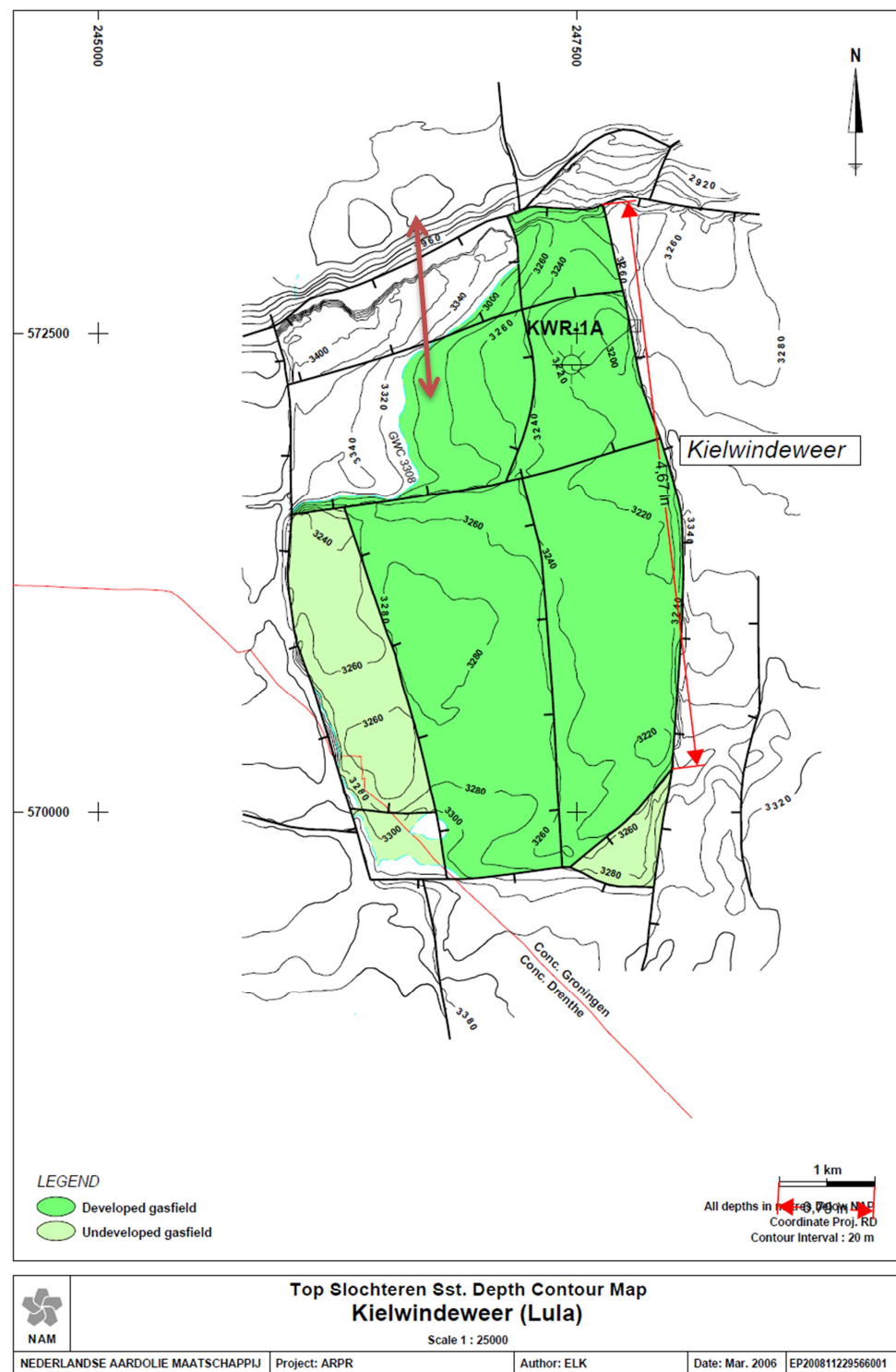
Figuur II.1 Structuurkaart van het Kiel-Windeweer veld (Winningsplan Kiel-Windeweer, NAM 2003). De diepte contourlijnen representeren de top van de Slochteren Formatie.
