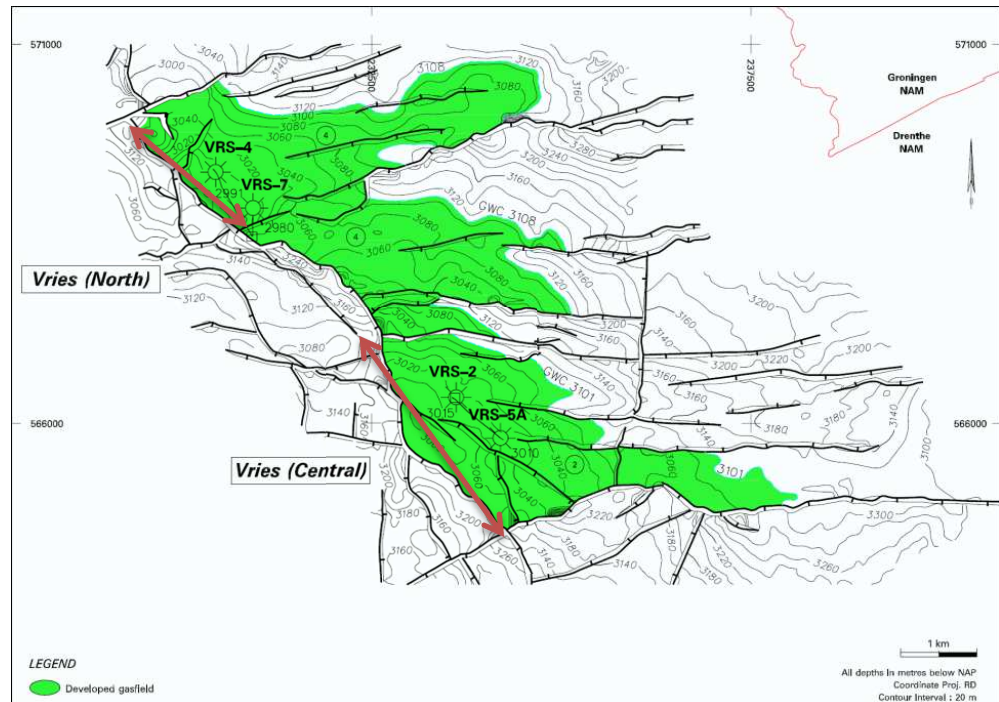
Figuur WWW.2 Structuurkaart van het Vries-North en -Central voorkomen (Winningsplan Westerveld, NAM 2003). De Boven-Rotliegend Groep vormt hier het reservoirgesteente.
