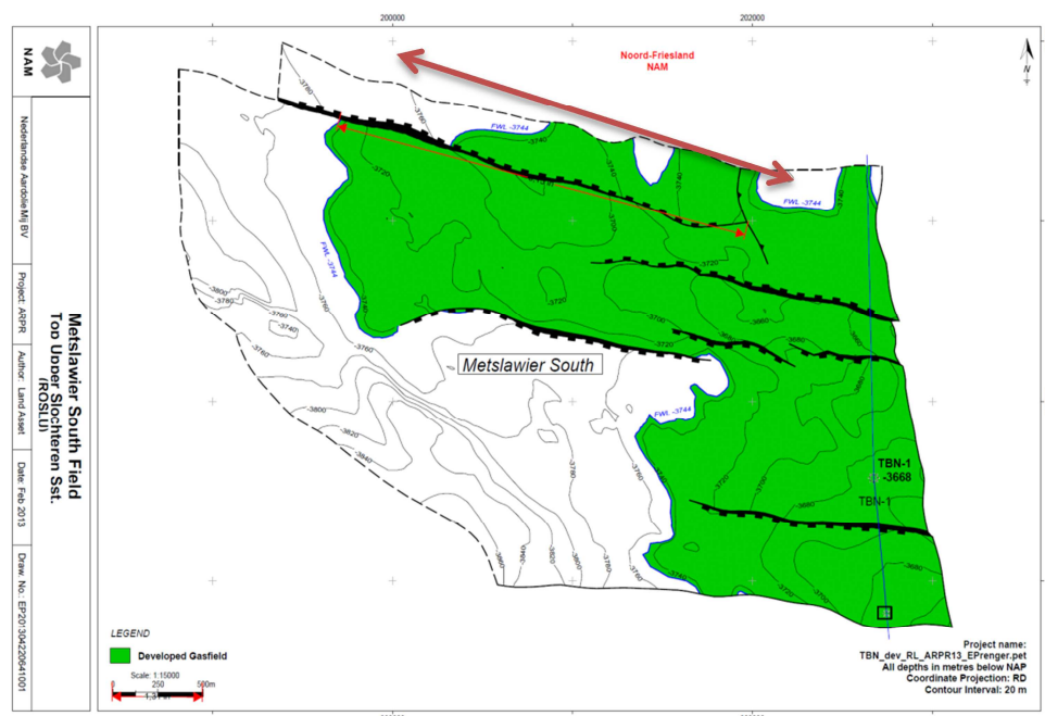
Figuur RR.1 Structuurkaart en doorsnede van het Metslawier-Zuid gasveld (Winningplan Metslawier-Zuid, NAM 2014).
