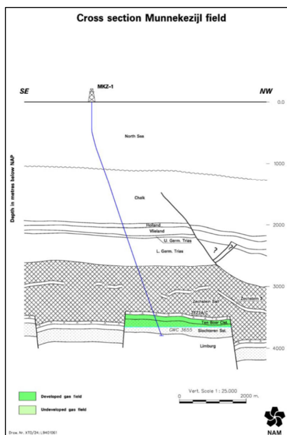
Figuur WW.2 Doorsnede van het Munnekeziel gasveld (Winningsplan Munnekeziel, NAM 2012).
