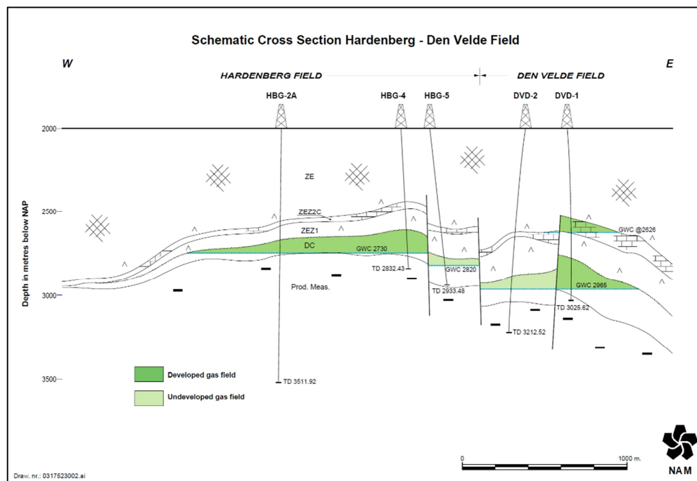
Figuur GG.2 Dwarsdoorsnede door het Hardenberg veld (Winningsplan Hardenberg-Oost, NAM 2013).
