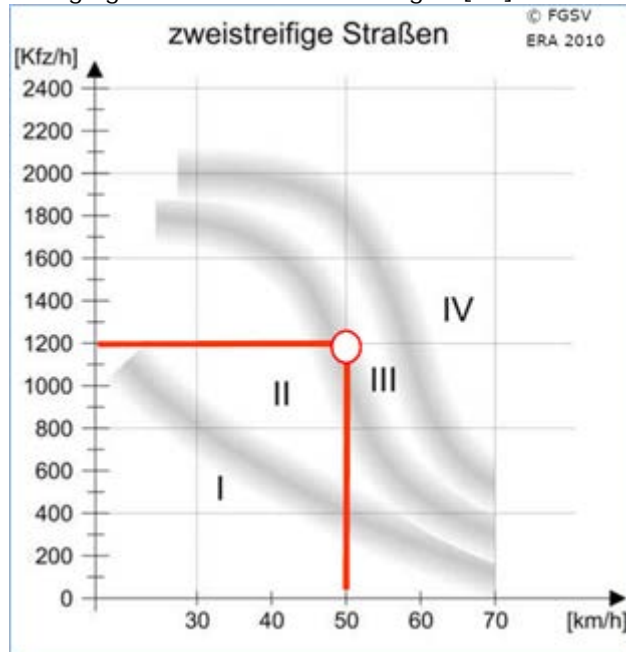
Afwegingsschema fietsvoorzieningen [22]
