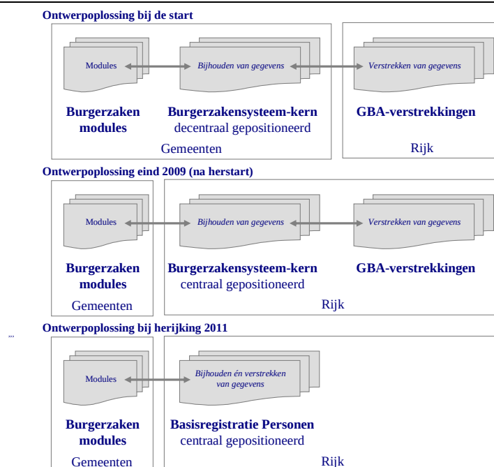
Figuur 3 : Ontwikkeling oplossingen voor de gemoderniseerde Gemeentelijke Basisadministratie (versimpelde weergave)
