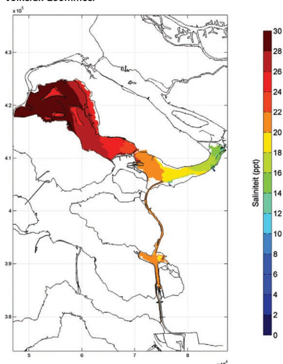
Figuur 31. Verspreiding van het zoete water uit het Hollands Diep en de Brabantse rivieren in de bovenste waterlaag van het Volkerak-Zoommeer en de Grevelingen; gehalten worden 50% van de tijd onderschreden (saliniteit = 1,2 x chlorositeit). Bron: Verwachte waterkwaliteit in een verbonden en zout Grevelingen – Volkerak-Zoommeer met getij – Deltares 2013.
