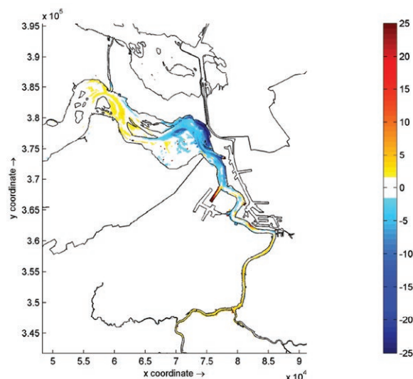
Figuur 44. Absoluut verschil (mg/l) in tijdgemiddelde slibconcentratie aan de bodem T1-To. Bron: Deltares 2014.
