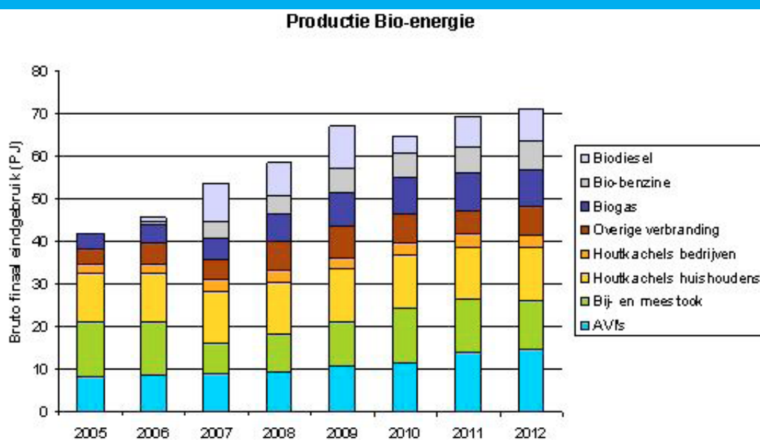
Figuur 1. Ontwikkeling van Bio-energie [PJ] uit verschillende bronnen in Nederland (2005 – 2012). AVI = afvalverbrandingsinstallatie
