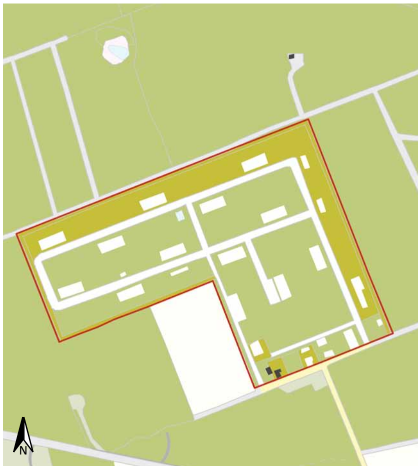
Plattegrond
