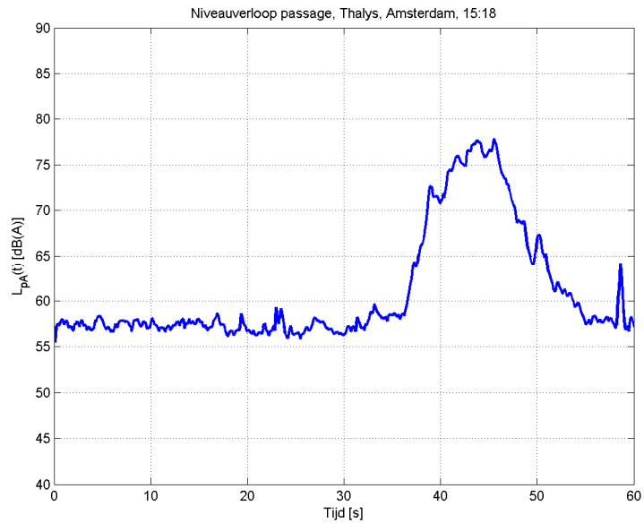
Figuur B1 Niveauperloop van de A-gewogen geluidniveau naast de woning aan de Fransche Brug 16 van een Thalys passage, richting Amsterdam, op 10 januari 2013 om 15:18.
