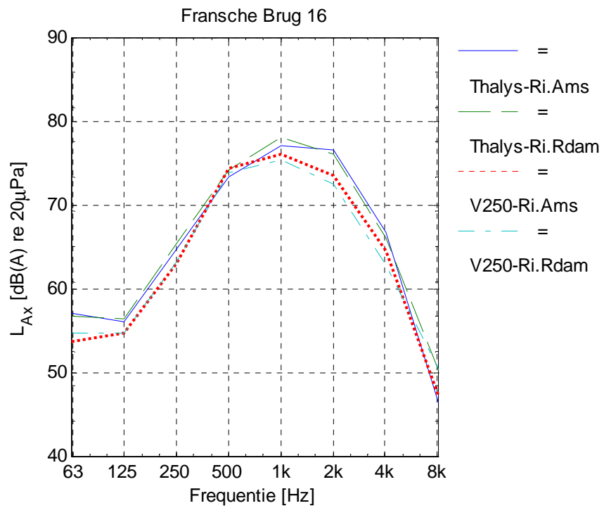
Figuur 12 Gemeten gemiddeld A-gewogen geluidexpositieniveaus L_{Ax} (dB(A) re. 20 \mu Pa), in octaafbanden, bij de woning aan de Fransche Brug 16, van alle geanalyseerde treinpassages van de Thalys en Ansaldo V250 per rijrichting.
