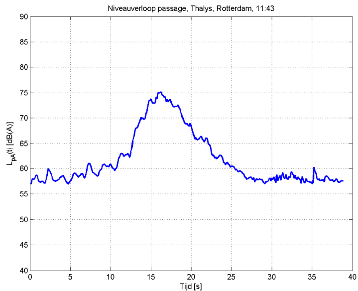
Figuur B2 Niveauperloop van de A-gewogen geluidniveau naast de woning aan de Fransche Brug 16 van een Thalys passage, richting Rotterdam, op 10 januari 2013 om 11:43.
