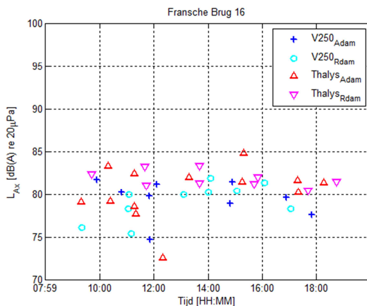
Figuur 11 Overzicht van de A-gewogen geluidexpositieniveaus ( L_{Ax} in dB(A) re. 20 \mu Pa) van de geanalyseerde geluidmetingen voor de gevel van de woning aan de Fransche Brug 16.
