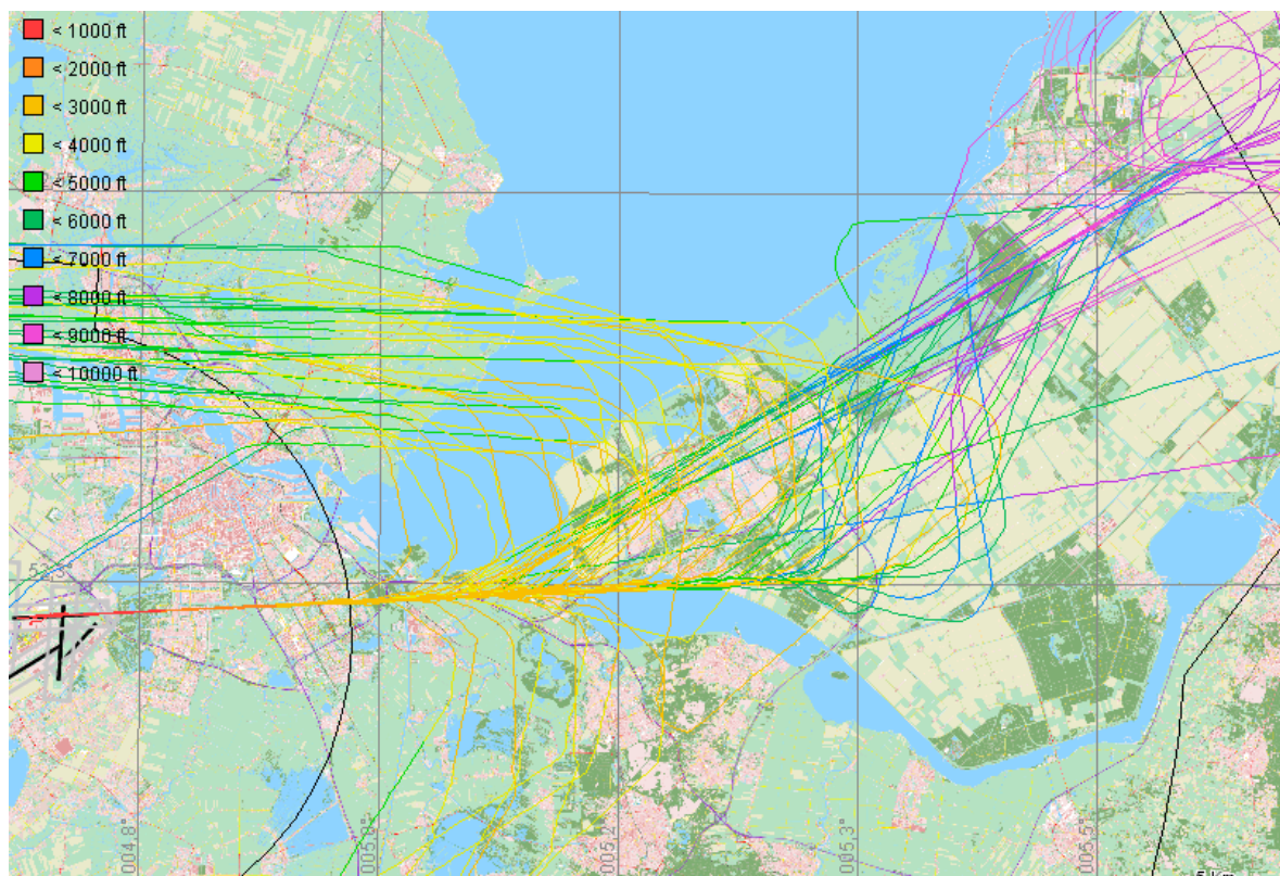
Figuur 23: Vectorpatronen Schiphol-verkeer bij landen 27 (Buitenveldertbaan) als enige landingsbaan bij harde westenwind (72 vluchten tussen 6.00 - 9.00 u LT op 9 december 2011).
