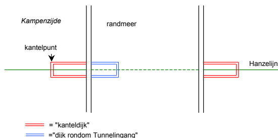
Figuur 34: Principe van de Kanteldijk
