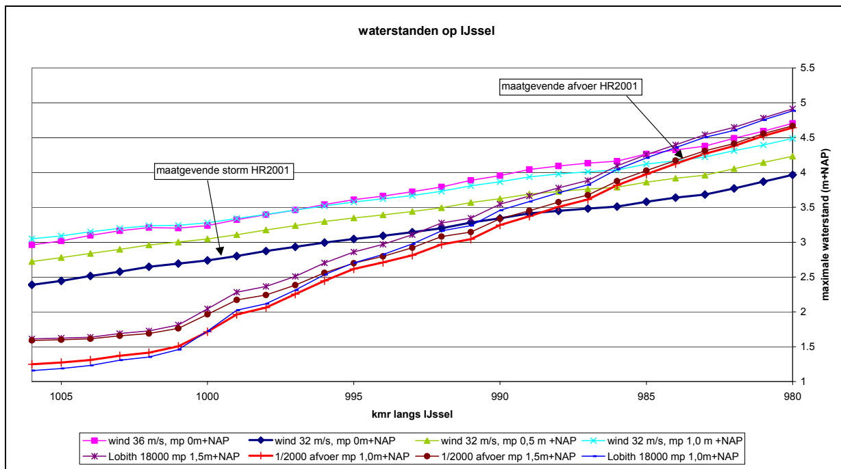
Figuur 17: Gevoeligheid voor klimaatscenario's op de IJssel
