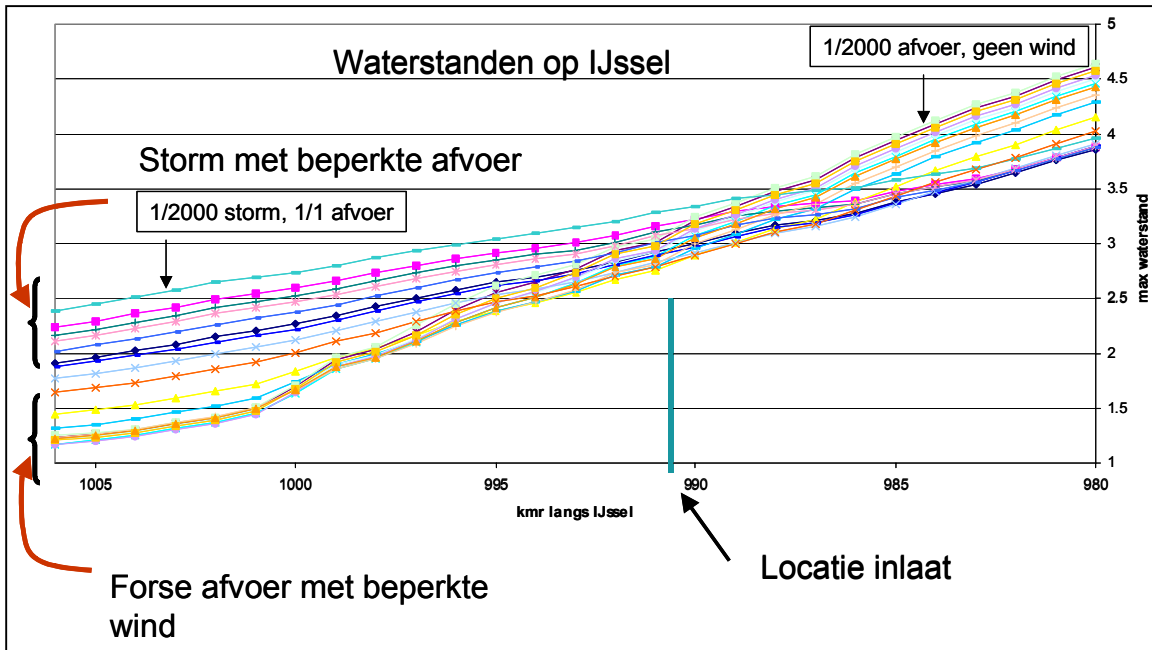
Figuur 13: Waterstanden bij verschillende combinaties op de IJssel
