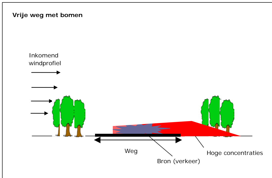
Figuur 16 Schematisch stromingspatroon bij een vrij liggende weg met bomen.
