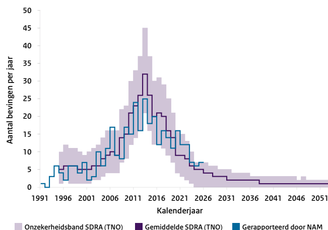
Figuur 4.3: Het aantal bevingen met een magnitude van 1,5 of groter per jaar in het Groningen-gasveld en omliggende aquifers zoals gerapporteerd door de NAM (blauwe lijn), en zoals voorspeld met de seismische dreiging- en risicoanalyse (SDRA) van de Nederlandse organisatie voor toegepast wetenschappelijk onderzoek (TNO, donkerpaarse lijn) met onzekerheidsband (lichtpaarse band). De bevingen vallen binnen de voorspelde bandbreedte. De NAM rapporteert alleen bevingen die ook met twee decimalen achter de komma een magnitude boven de 1,5 hebben en rond dus een bijvoorbeeld een magnitude 1,49 beving niet af naar boven. De beving bij Warffum op 18 mei 2025 is ook meegenomen in dit figuur omdat een verband met het Groningen-gasveld niet valt uit te sluiten.
