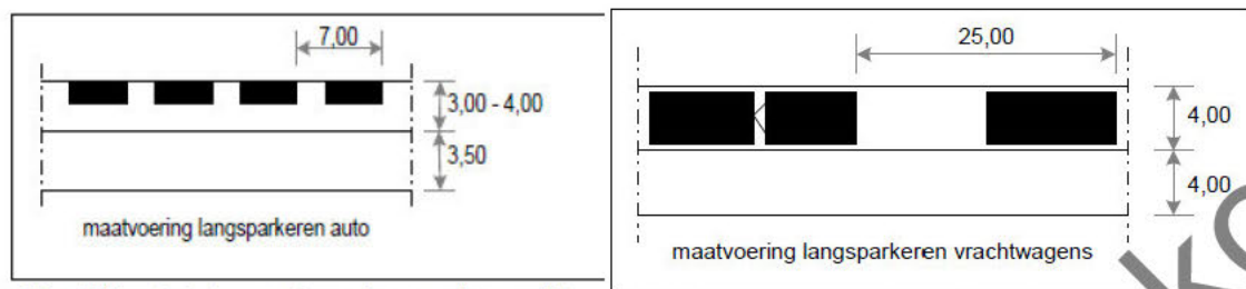
Afbeelding 5.1.1: maatvoering parkeervakken
