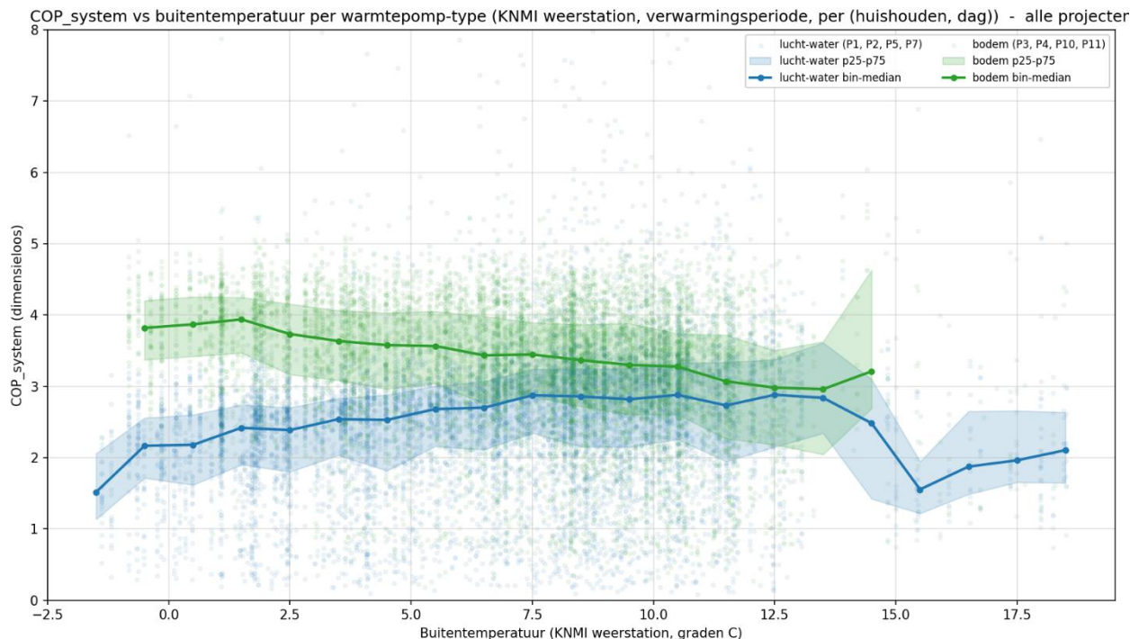
Figuur 14: Daggemiddelde COP's van woningen met een lucht-water (blauw) en bodem (groen) warmtepomp
