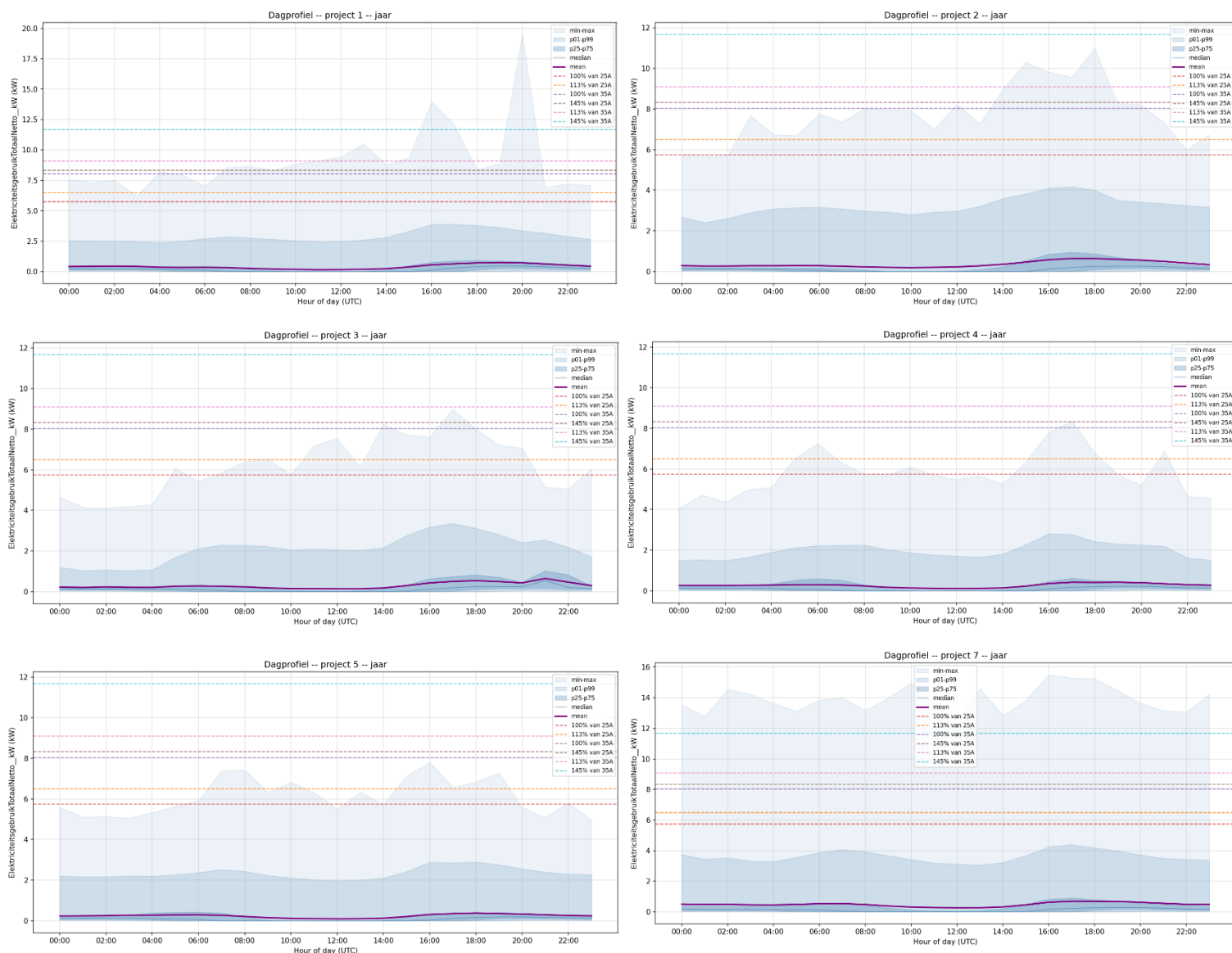
Figuur 12: Dagprofielen van projecten 1, 2, 3, 4, 5 en 7
