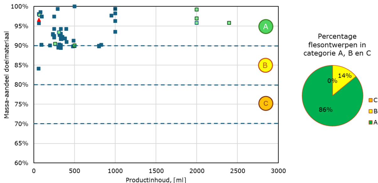
Figuur 2: Relatie tussen het productvolume van de zuivelfles en de recyclebaarheid in termen van het massa-aandeel doelmateriaal. De PET-flessen zijn weergegeven als donkerblauwe vierkantjes, de HPDE flessen als groene vierkantjes en de PS-flessen als rode driehoeken. NB. Dit gaat over de individuele flesontwerpen en niet over het marktaandeel. Rechts het aandeel flesontwerpen in iedere categorie.
