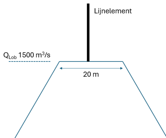
Figuur C.2: Boven: Dwarsdoorsnede langsamschematisatie welke overeenkomt met de schematisatie van de bestaande langsdommen.
