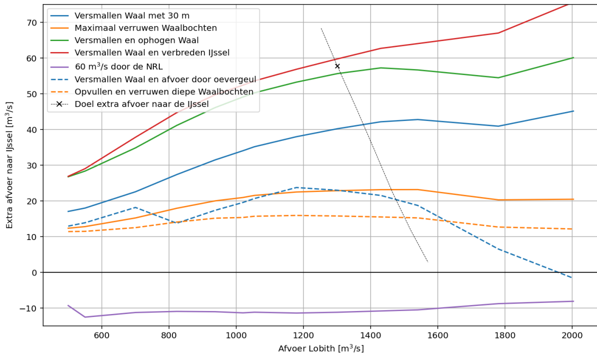
Figuur 5.1: Extra afvoer naar de IJssel als functie van afvoer bij Lobith.
