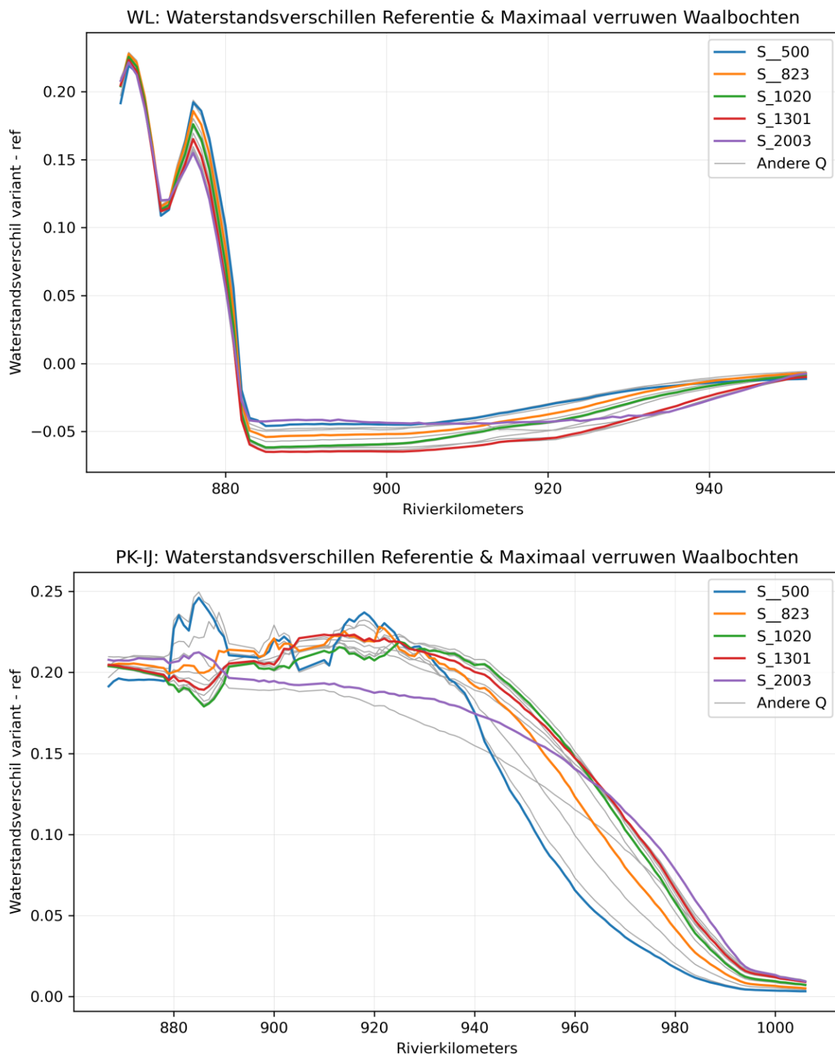
Figuur 3.13: Waterstandsverschillen ten opzichte van de referentiesituatie langs de Waal (boven) en het traject Pannerdensch Kanaal – IJssel.
