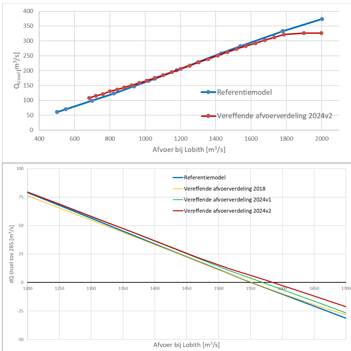
Figuur A.1: Boven: vergelijking IJsselaflow bij de vereffende afvoerverdeling 2024 v2 en de resultaten van het referentiemodel. Onder: vergelijking afvoerverschil IJssel t.o.v. 285 \text{m}^3/\text{s} voor de vereffende afvoerverdelingen 2018, 2024 v1, 2024 v2 en het referentiemodel
