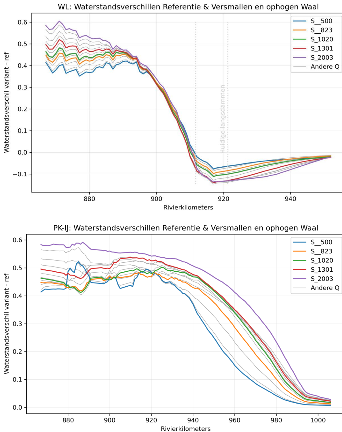
Figuur 3.7: Waterstandsverschillen ten opzichte van de referentiesituatie langs de Waal (boven) en het traject Pannerdensch Kanaal – IJssel.
