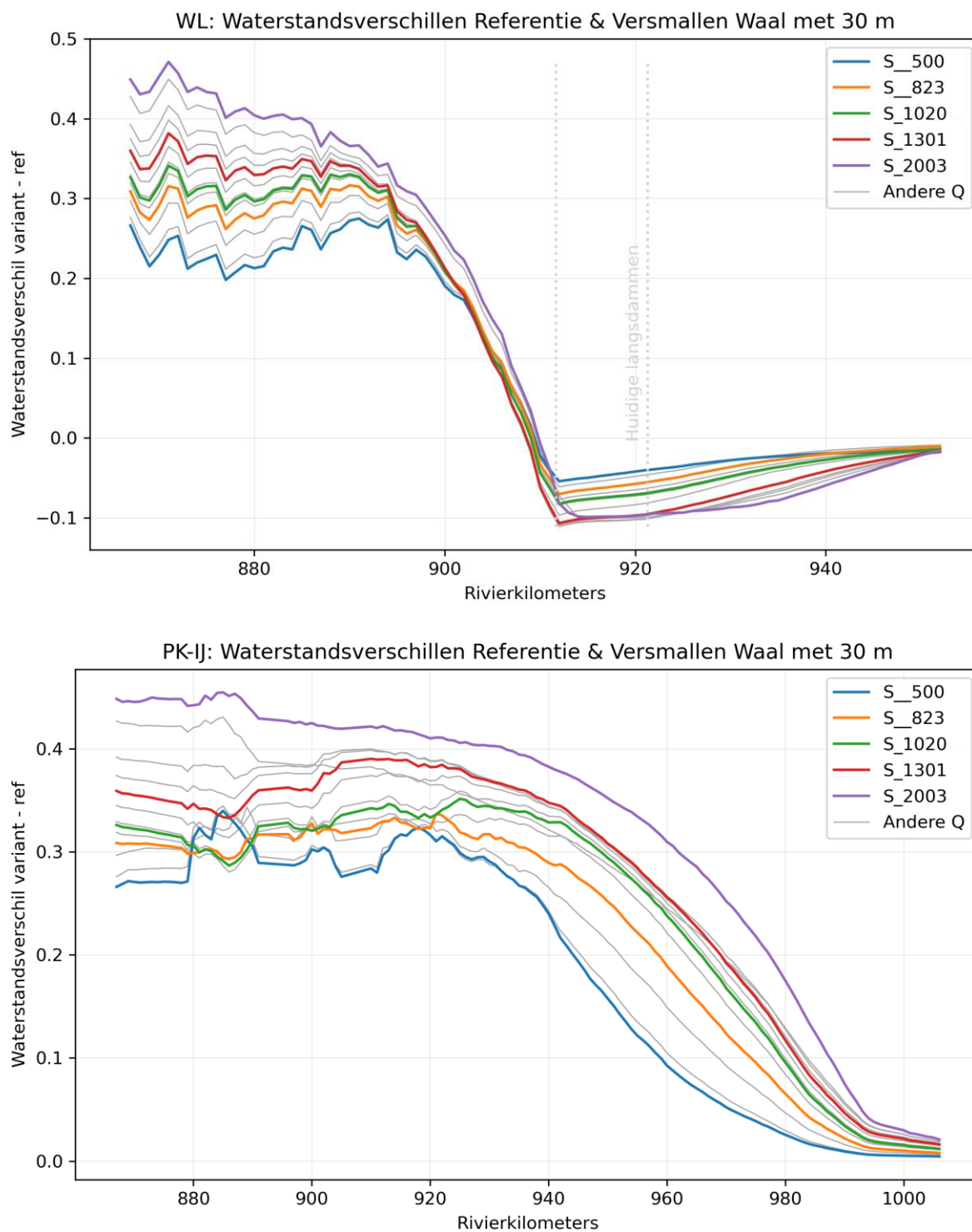
Figuur 3.4: Waterstandsverschillen ten opzichte van de referentiesituatie langs de Waal (boven) en het traject Pannerdensch Kanaal – IJssel.
