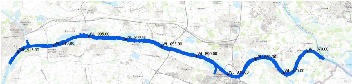
Figuur 3.5: Traject waarop de verhoging van de Waalbodem wordt toegepast.
