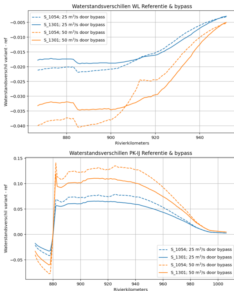
Figuur 4.12: Waterstandsverschillen ten opzichte van de referentiesituatie langs de Waal (boven) en het traject Pannerdensch Kanaal – IJssel.
