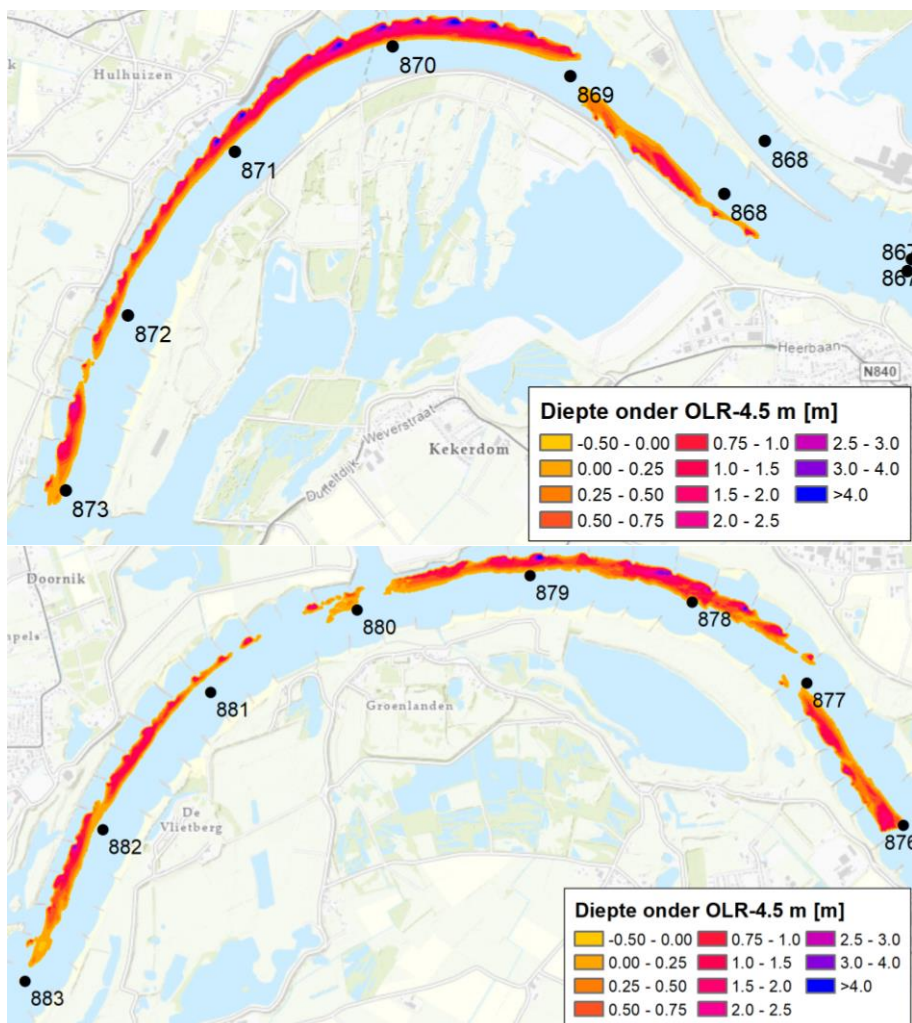
Figuur 4.8: De vlakken waarin de bodemhoogte in de Waalbochten lager ligt dan OLR-4,5 m waarbij de kleurschaal aangeeft hoe ver de bodem onder OLR-4,5 m ligt. Deze vlakken worden opgehoogd tot het niveau van OLR-4,5 m.
