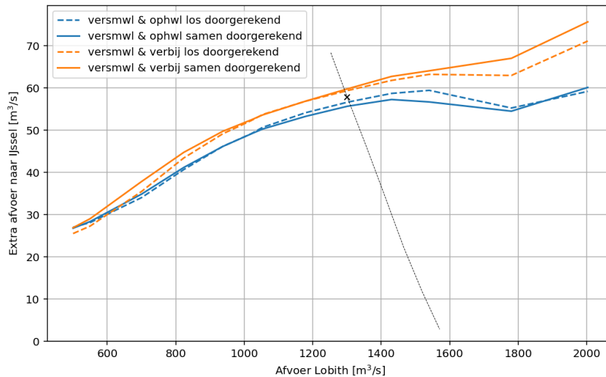
Figuur 4.1: Optelbaarheid van los doorgerekende maatregelen voor de maatregelen versmallen Waal in combinatie met ophogen van de Waalbodem (blauw) en verbreden van de IJssel (oranje).
