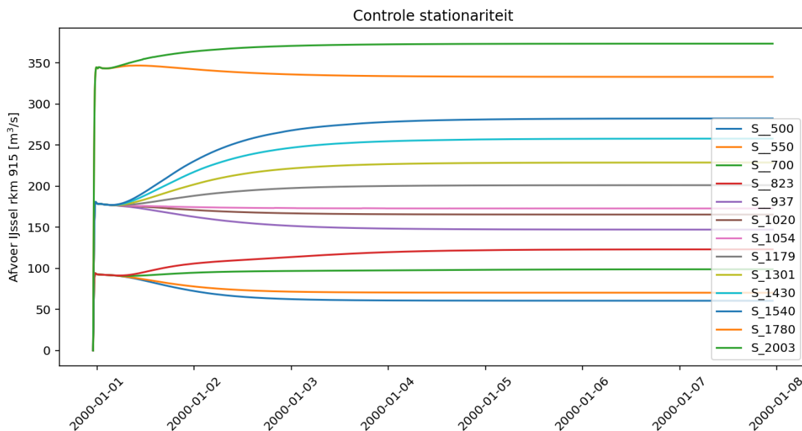
Figuur 2.1: Controle op stationariteit van de referentieberekeningen door het weergeven van de IJsselafoeren op rivierkilometer 915,47.
