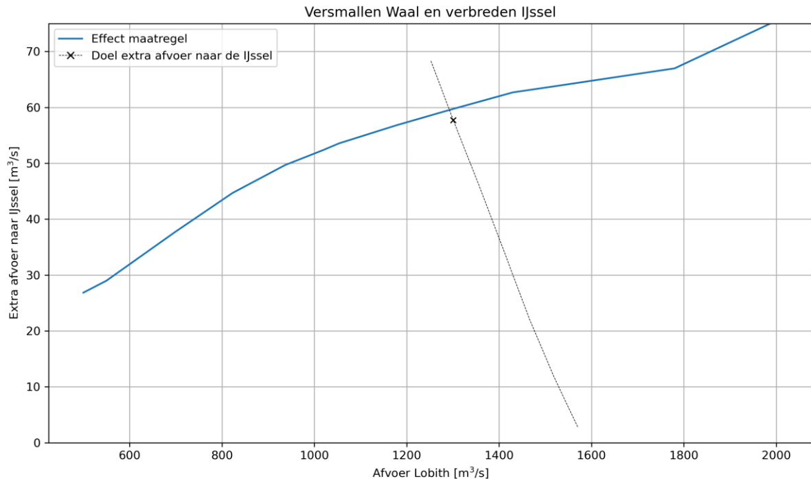
Figuur 3.9: Effect van een versmalling van de Waal en een verbreding van de IJssel op de afvoer naar de IJssel als functie van Lobithafvoer.
