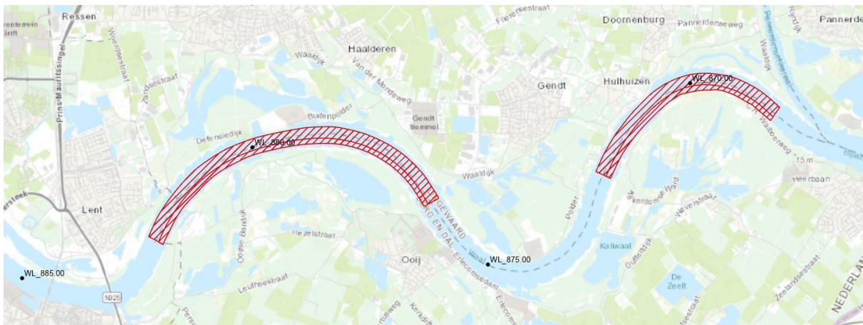
Figuur 3.11: Trajecten waarop de buitenbocht is verruwd. De verruwing wordt toegepast op 2/3^e van de breedte van het zomerbed.
