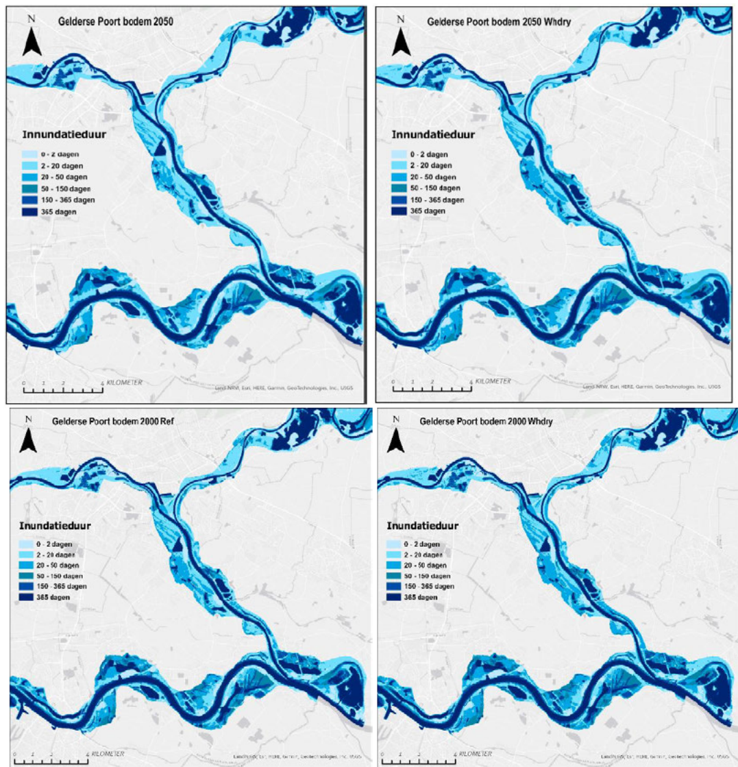
Figuur 6-3 Overstromingsduur van de uiterwaarden in de Gelderse Poort bij verschillende rivierbodempliggingen (boven in het jaar 2050, onder rond het jaar 2000) en klimaat (links het huidige klimaat, rechts WHdry). Het verschil in bodempligging was maximaal ~80 cm op de Boven-Waal, wat zich vertaalde in een waterstandsverschil van 50 cm bij lage afvoeren afnemend tot 20 cm bij hoge afvoeren. In deze figuren is geen rekening gehouden met zomerkades (bron: Asselman et al., 2022a,b).
