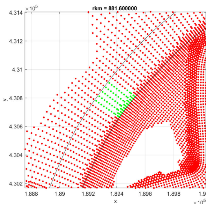
Figuur 3-5 Voorbeeld van een 200 m lang vak langs de Waal. Met groene stippen gemarkeerde roosterzellen worden gebruikt voor de middeling van de stroomsnelheid en de sedimentsamenstelling voor het vak rond rkm 881,6. Deze rivierkilometer ligt in het midden van het vak.
