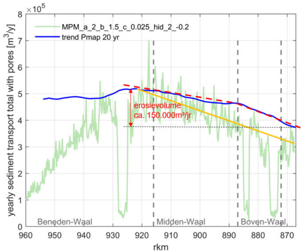
Figuur 5-3 Jaarlijks sedimenttransport (inclusief poriën) geschat volgens de in voorliggend rapport beschreven methode (groene lijn) en geschat uit de trends in bodemverandering in de afgelopen 20 jaar van Sloff (2019) (blauwe lijn). De rode streepjeslijn geeft een schatting van het jaarlijks erosievolume dat gecompenseerd moet worden om de bodemligging constant te houden. De doorgetrokken oranje lijn geeft aan hoe groot dit volume volgens de in dit rapport gebruikte methode zou zijn. De gesuggereerde zeer lage transporten op de drie trajecten met vaste lagen en als vaste lagen geschematiseerde bodemkribben vormen modelartefacten als toegelicht in paragraaf 5.2.
