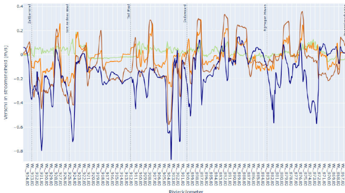
Figuur 4-11 Verschil in stroomsnelheid tussen de referentie en de uiterwaardegeulvariant bij vier afvoeren: 1020 m 3 /s (groen), 2020 m 3 /s (oranje), 5800 m 3 /s (bruin) en 16.000 m 3 /s (paars). Weergegeven is het deel van de Waal waar de geulen zijn toegepast (Pannerdensche Kop – Zaltbommel). De volledige figuur is opgenomen in bijlage B.3.
