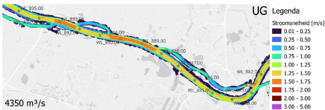
Figuur 4-15. Stroomsnelheden bij 4350 m³/s in de UG-variant ter hoogte van Nijmegen.
