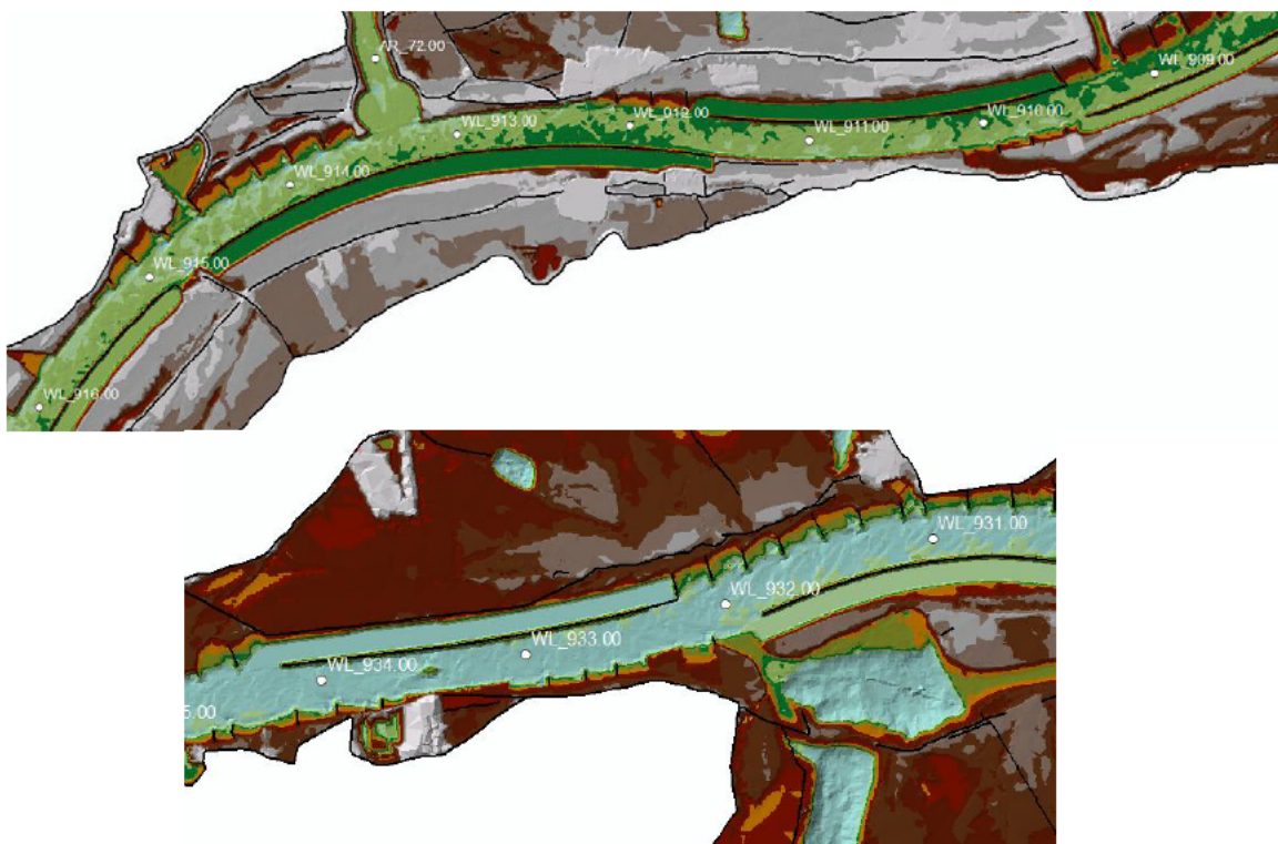
Figuur 5-12 Locaties waar de bodemligging in de oevergeulen duidelijk afwijkt van de geul boven- of benedenstrooms ervan. De geul die bij rkm 932 start begint op een bodemhoogte van -3,30 m +NAP, terwijl het einde van de voorgaande geul op -2,60 m +NAP ligt.
