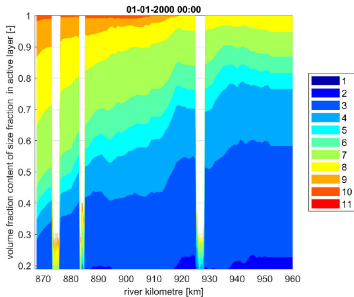
Figuur 3-3 Sedimentsamenstelling uit het DVR-model. De kleurschaal toont de verdeling in sedimentklassen (zeefklassen) zoals gedefinieerd in Tabel 3-3.
