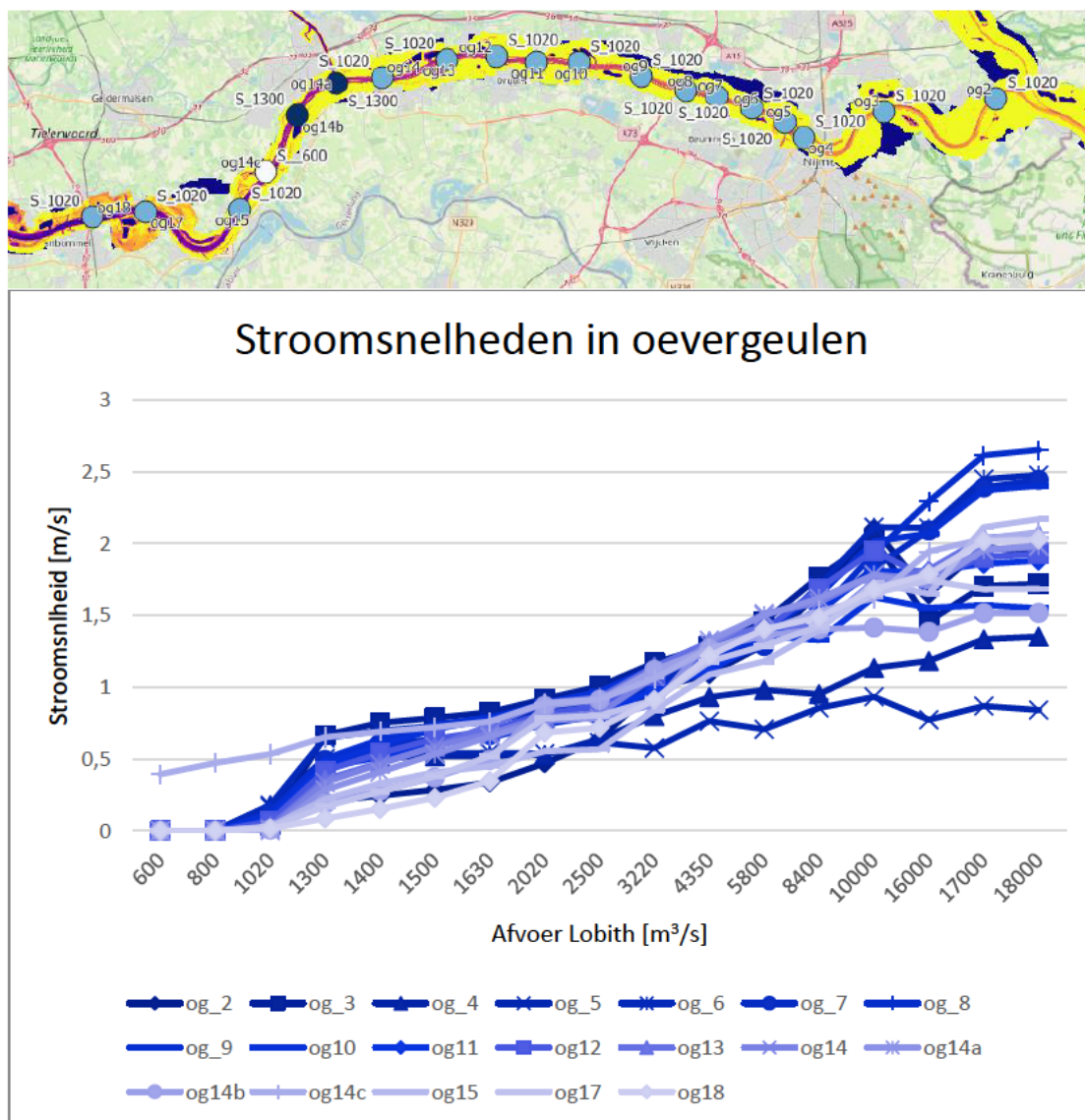
Figuur 4-16 Boven: De ligging van de oevergeulen en de afvoer waarbij deze mee beginnen te stromen. Onder: Stroomsnelheden in de oevergeulen bij de doorerekende afvoeren. De kleuren worden lichter in de stroomafwaartse richting
