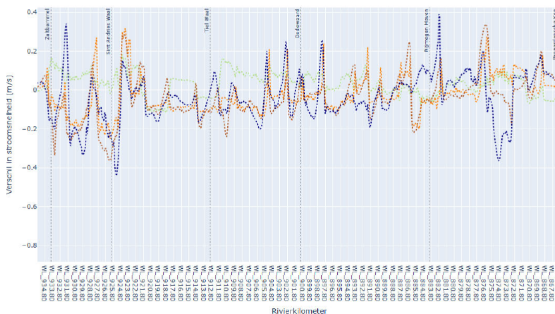
Figuur 4-12 Verschil in stroomsnelheid tussen de referentie en de oevergeulvarianten bij vier afvoeren: 1020 m 3 /s (groen), 2020 m 3 /s (oranje), 5800 m 3 /s (bruin) en 16.000 m 3 /s (paars). Weergegeven is het deel van de Waal waar de geulen zijn toegepast (Pannerdensche Kop – Zaltbommel). De volledige figuur is opgenomen in bijlage B.3.
