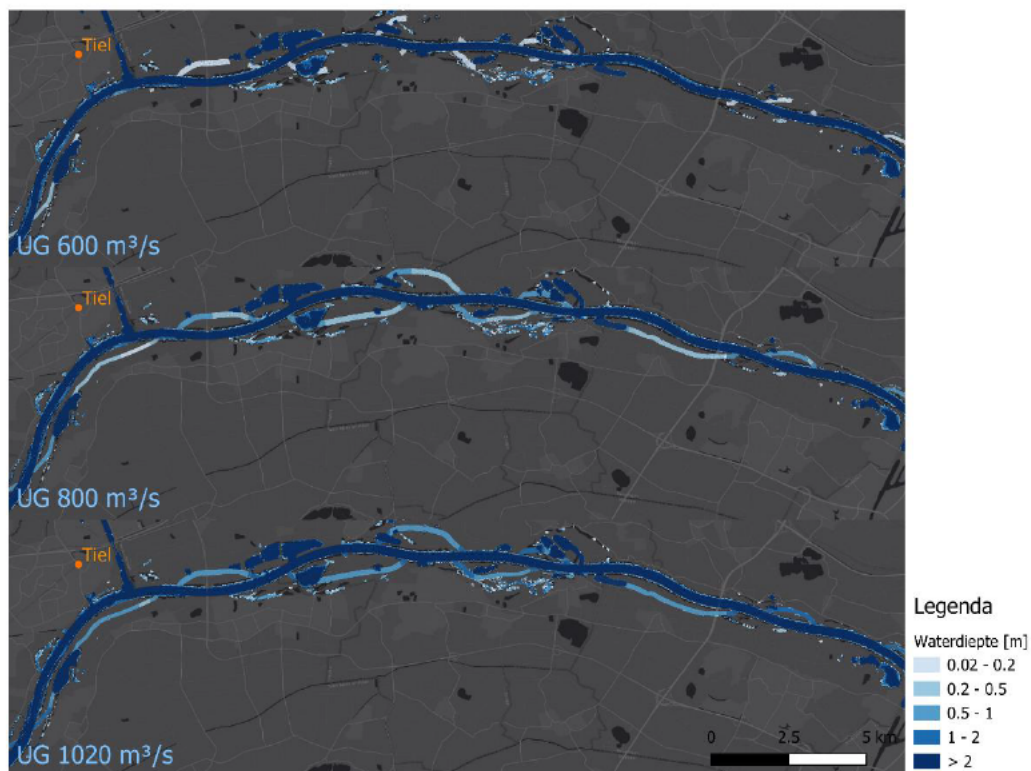
Figuur 6-2. Waterdiepte bij lage afvoeren (600, 800 en 1020 m 3 /s) in de UG-variant.
