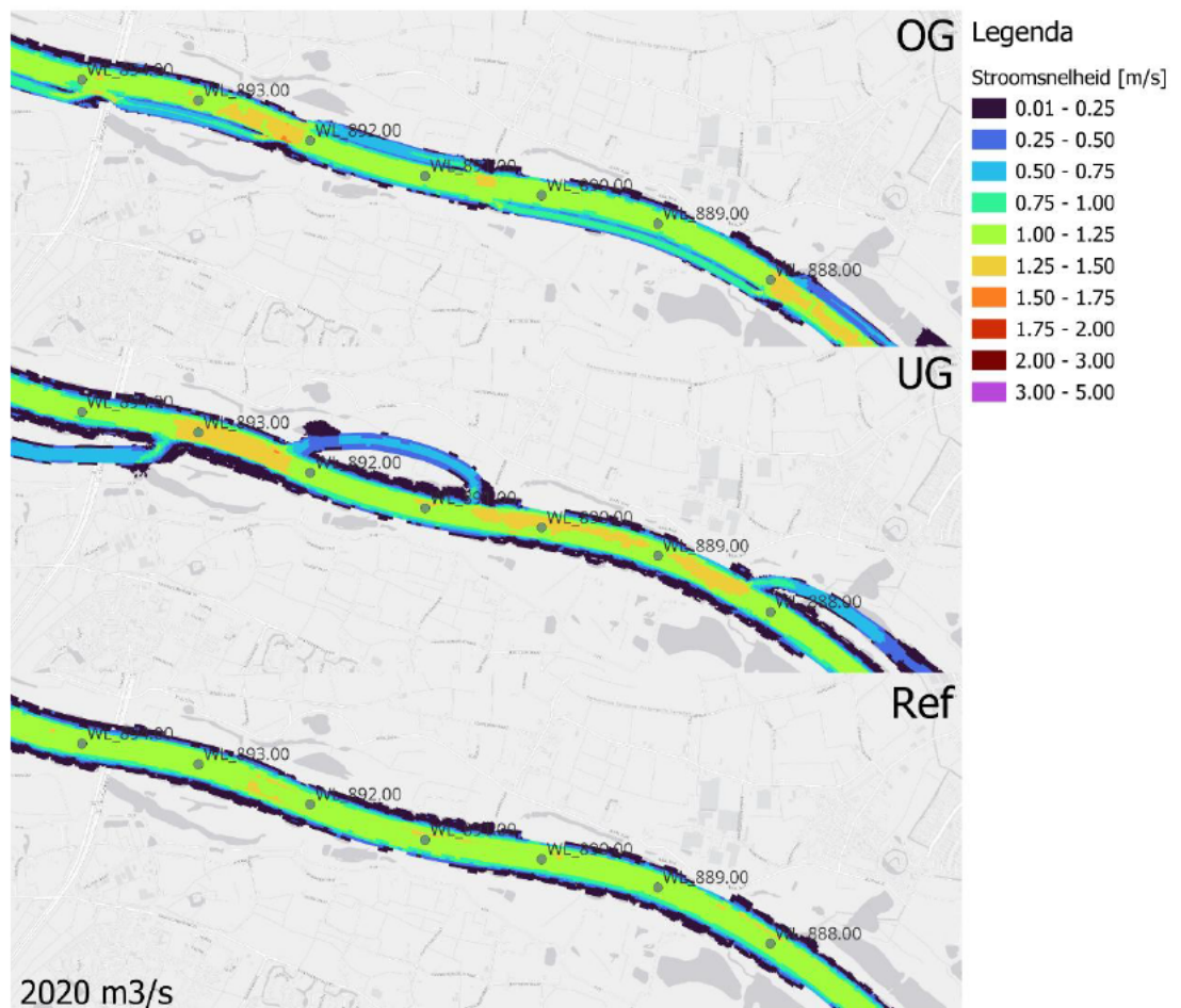
Figuur 6-5. Stroomsnelheden in de verschillende varianten bij een afvoer van 2020 m³/s bij Lobith.
