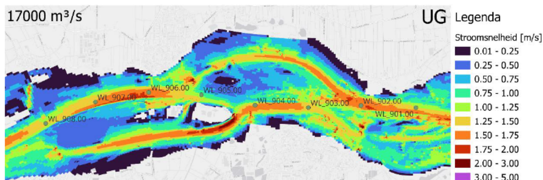
Figuur 4-13 Ruimtelijke variatie in stroomsnelheid bij een afvoer van 17.000 m 3 /s ter hoogte van Druten waar overlappende uiterwaardgeulen zijn geschematiseerd in het model.
