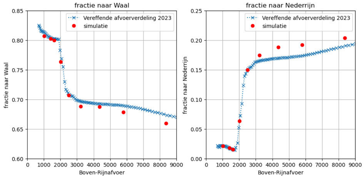
Figuur 3.2 Afvoerdeling bij de splitsingspunten op basis van de vereffende afvoerdeling 2023 en het referentiemodel.
