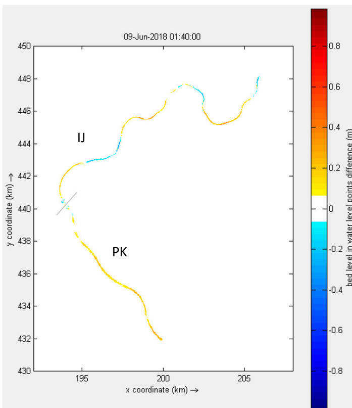
Figuur 5.21 MP4 – aansluiten Zwarte Schaar: Vershil in bodemligging met referentie na 20 jaar morfologische ontwikkeling voor Pannerdensch Kanaal en Boven-IJssel (tot brug Doesburg).
