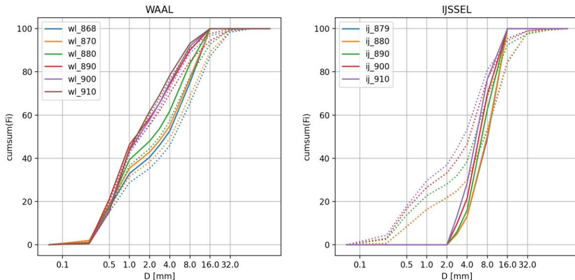
Figuur 4.3 De korrelgrootteverdeling van de suppleties in de Waal en de IJssel per 10 km (gestippelde lijnen) en die van de suppletie. In de Waal zijn geen mobiele sedimentklassen meegenomen, waardoor het suppletiemateriaal fijner is dan het lokale bodemmateriaal. In de IJssel moet relatief grof materiaal gesuppleerd worden (zie paragraaf 4.2.1) en daarom zijn de zandklassen weggelaten. Daarnaast zijn ook de mobiele sedimentklassen weggelaten.
