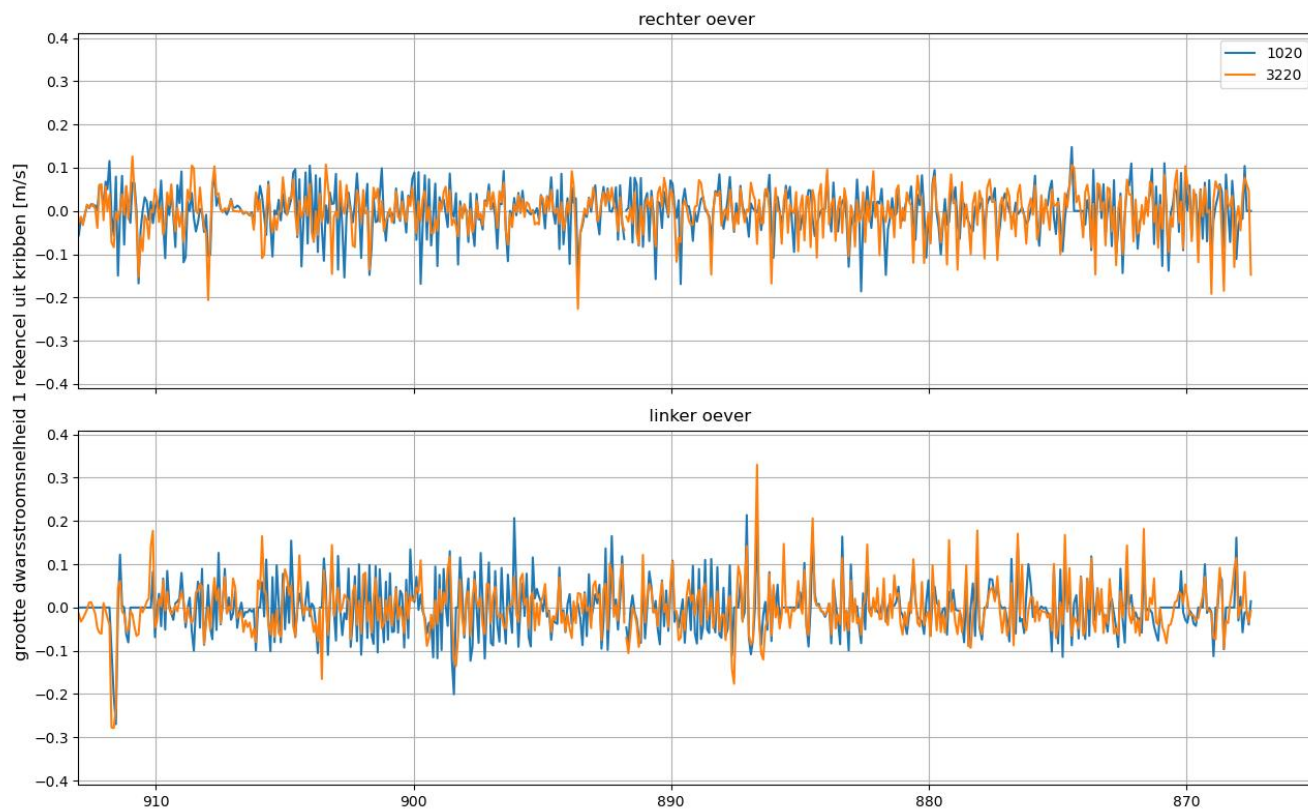
Figuur 9.12 Inschatting dwarsstroming in referentie (initieel) (M-lijnen 15 en 25). Stroming in dit figuur is van rechts naar links
