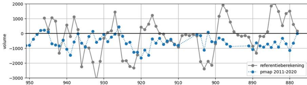
Figuur 4.4 Volume horende bij de bodem per jaar in de IJssel volgens de referentieberekening en de PMAP-trend. Een negatief volume is gelijk aan een benodigd suppletievolume. Een positief volume is sedimentatie.
