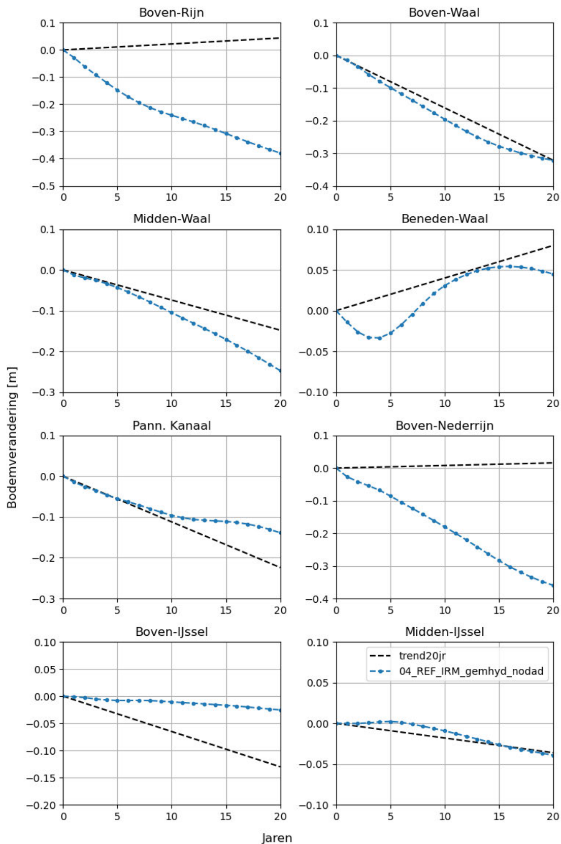
Figuur 3.3 Gemeten bodemtrends per riviervoorbeeld over 20 jaar (Tabel 2.1) vergeleken met de bodemtrends in het referentiemodel (04_REF_IRM).
