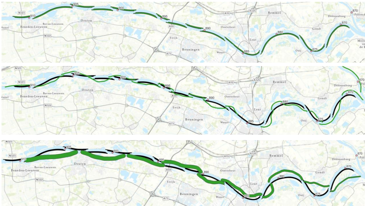
Figuur 7.4 Indicatieve schets van de vormgeving van het meergeulenconcept met diepe oevergeulen zoals toegepast in dit onderzoek (boven), dimensionering met nevengeulen gebaseerd op de visie 'Ruimte voor Middenafvoeren' van het WWF (midden) en een ontwerp met ondiepe, langere en brede nevengeulen, vermoedelijk nodig om de bodemerrosie te stoppen (onder).
