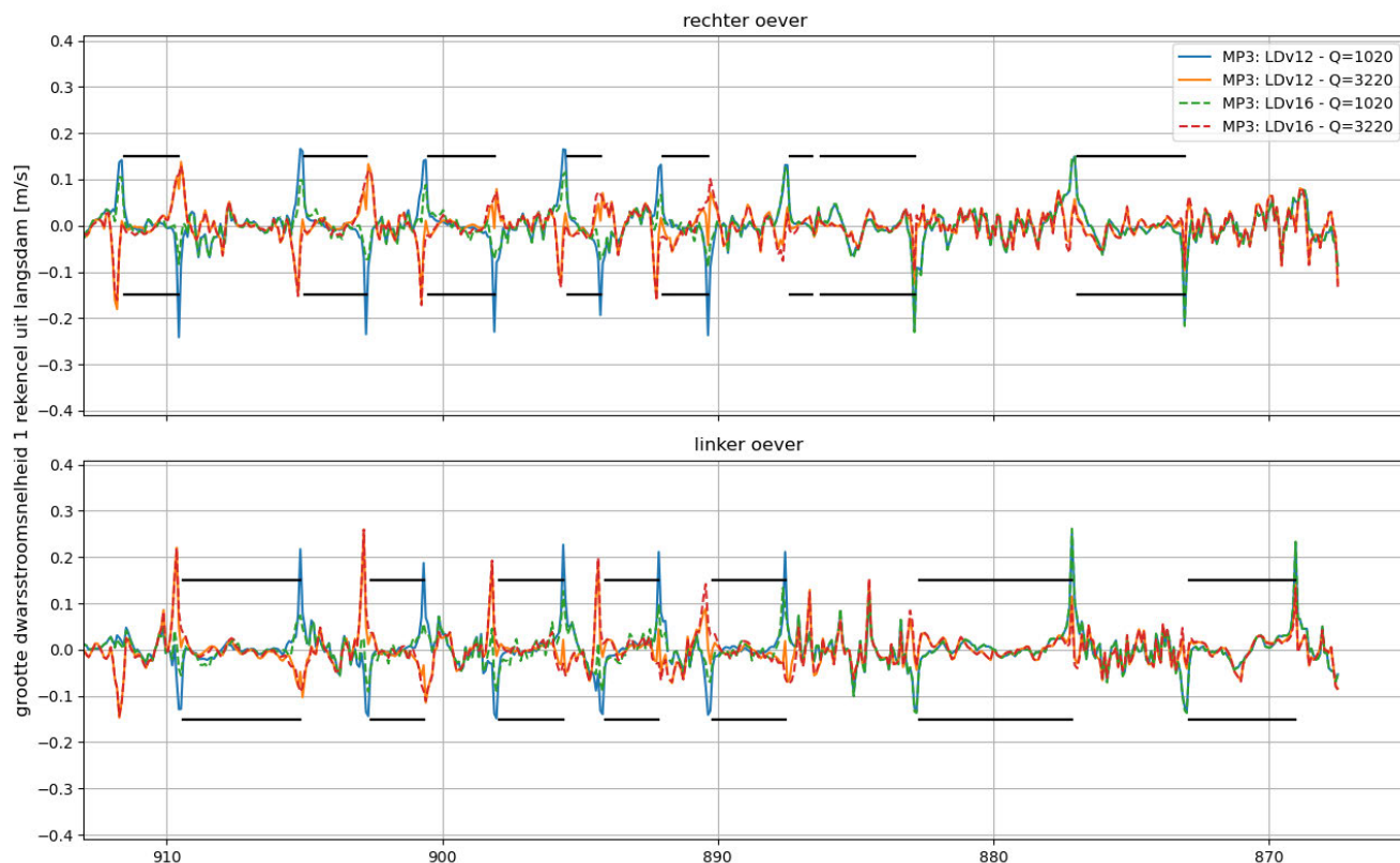
Figuur 9.11 Inschatting dwarsstroming voor MP3 (initieel) (M-lijnen 17 en 23). De horizontale zwarte lijnen geven locaties van langsdammen aan. Stroming in dit figuur is van rechts naar links.
