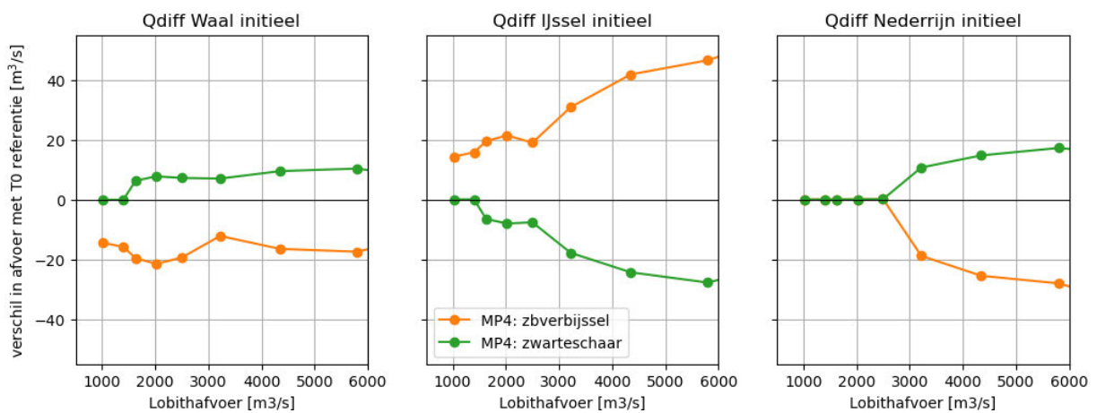
Figuur 4.13 Initieel effect op de IJsselaflow (midden) van de verbreding van de Boven-IJssel en van de aansluiting van het Zwarte Schaar bij de morfologische afvoersteps.
