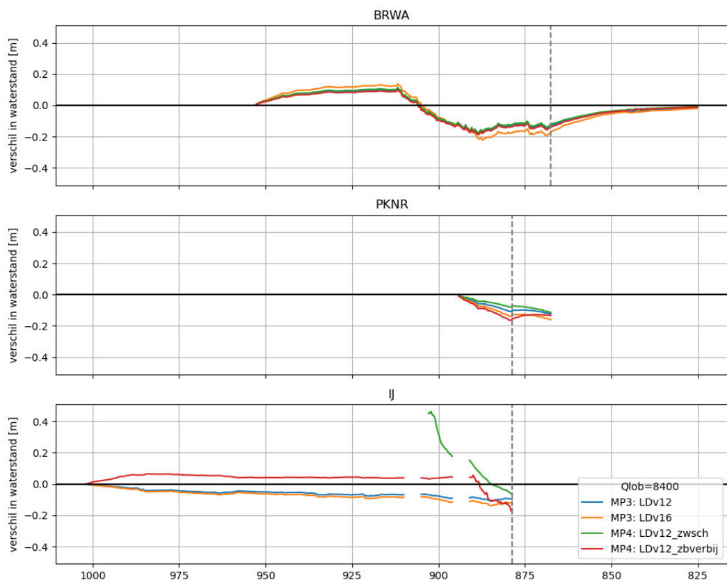
Figuur 9.8 Initieel effect op de waterstand bij Q8400 voor maatregelpakketten waarbij de riviergeometrie initieel wordt aangepast.
