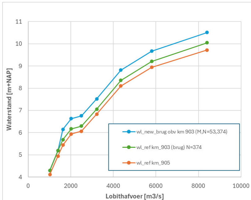
Figuur 4.16 Waterstandsrand bij de brug (ongeveer rkm 903) zonder (groen) en met (blauw) aansluiten het Zwarte Schaar.
