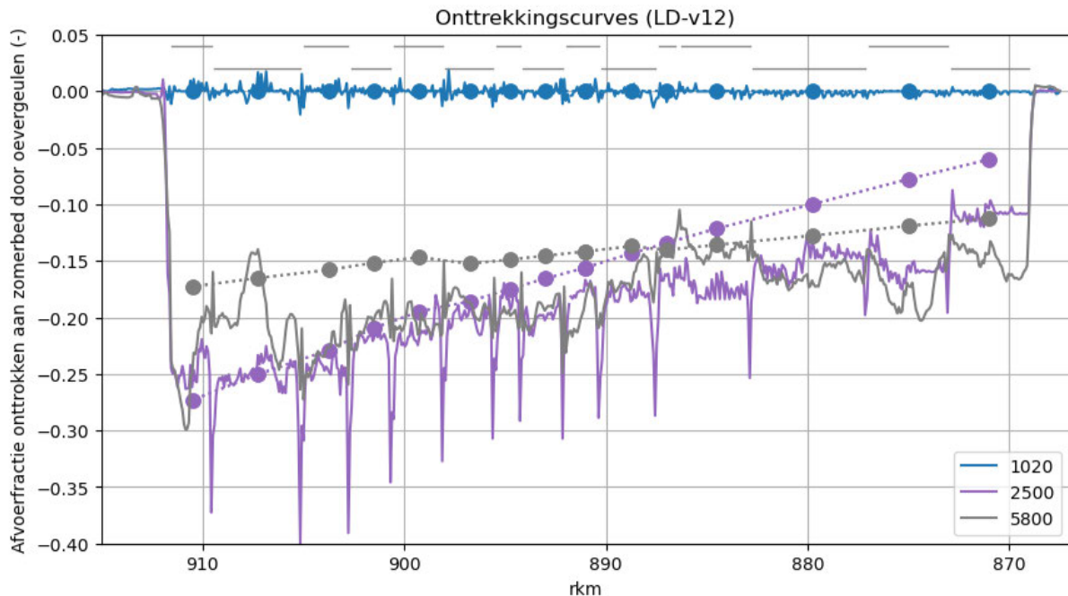
Figuur 7.2 Geschatte en berekende afvoeronttrekking aan de hoofdgeul door langsdammen (40 m versmalling) en oevergeulen bij drie afvoerniveaus op de Boven-Rijn. De geschatte afvoeronttrekkingen zijn bepaald met het evenwichtstool en weergegeven met stippellijnen en bolletjes.
