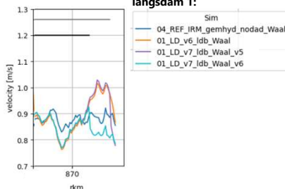
Stroomsnelheid bij Q1020 gaat omlaag bij verplaatsen start langsdam 1:
