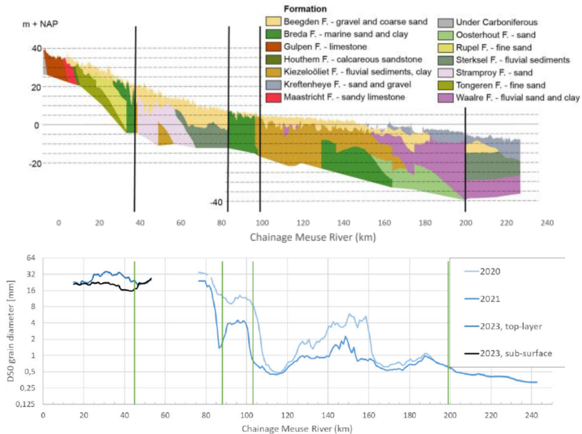
Figuur 8: Figuren uit Barneveld et al. (2025b). Boven: Langsprofiel van de bodemopbouw van de Maas. De zwarte lijnen geven de voor de riviermorphologie meest bepalende breuklijnen aan. Onder: de mediane korrelgrootte van de toplaag (in een deel van de Gemeenschappelijke Maas is er ook informatie van de laag eronder weergegeven) van de rivierbodembodem voor verschillende meetmomenten op basis van metingen van Rijkswaterstaat.
