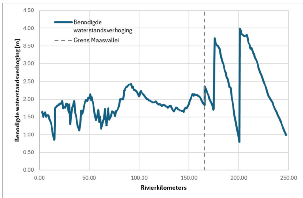
Figuur 59: Benodigde waterstandsverhoging om de inundatiefrequenties te verhogen naar de gekozen niveaus.
