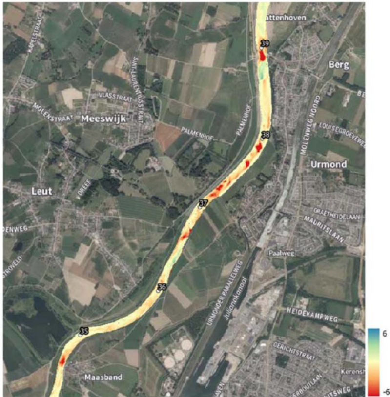
Figuur 20: Bodemhoogteverschil in het erosiekuilentrace voor en na het hoogwater van 2021. Figuur uit Expertisenetwerk (2021).
