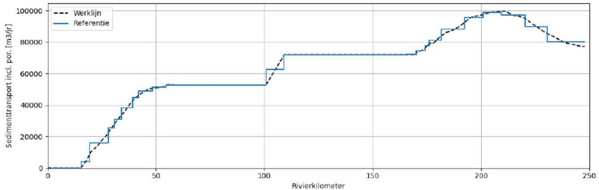
Figuur 56: Sedimenttransport langs de Maas: de vastgestelde werklijn en het gefitte model.
