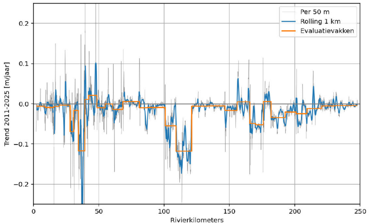
Figuur 49: Lineaire trends in gemiddelde rivierbodemligging per 50 m, per 1 km en in de evaluatievakken.
