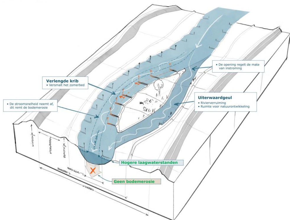
Figuur 2.9: Meergeulensysteem Waal – Variant uiterwaardgeul met verlengde kribben.
