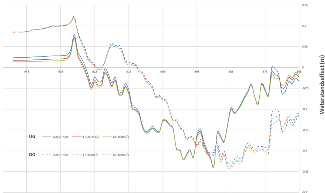
Figuur 2.16: Waterstandseffect op de Waal voor de Boven-Rijnafvoeren van 16.000, 17.000 en 18.000 m³/s voor de onderzoeksvarianten van het meergeulensysteem met oevergeulen en langsdammen (OG) en kribverlenging met uiterwaardgeulen (UG).
