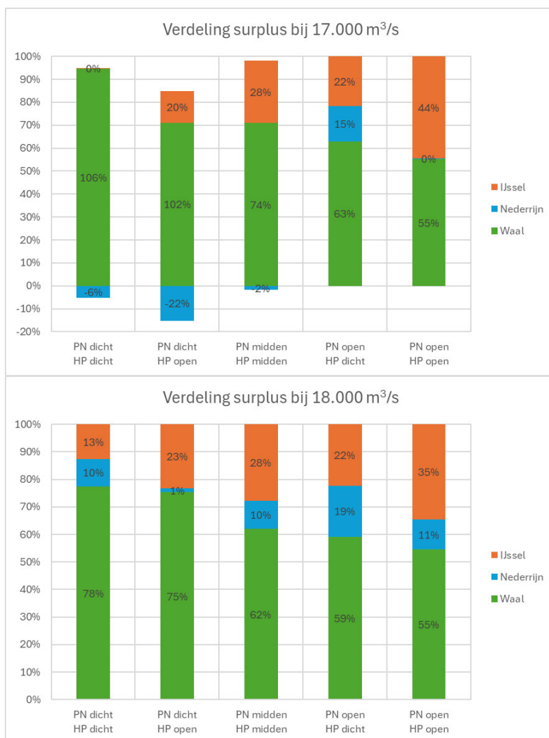
Figuur 2.7: Verdeling van het surplus bij 17.000 m³/s (boven) en 18.000 m³/s (onder) bij een riviergeometrie met oevergeulen en de regelwerken in de uiterste standen en de middenstand (PN = regelwerk Pannerden, HP = regelwerk Hondsbroeksche Pleij).
