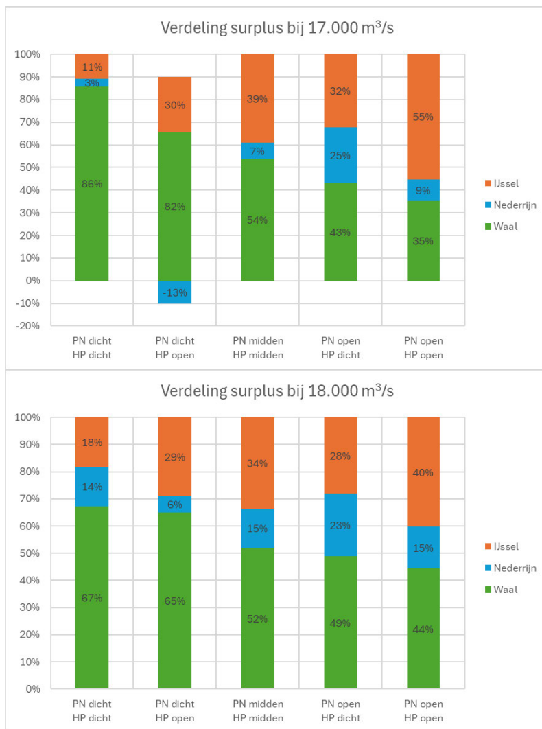
Figuur 2.6: Verdeling van het surplus bij 17.000 m³/s (boven) en 18.000 m³/s (onder) bij de huidige riviergeometrie en de regelwerken in de uiterste standen en de middenstand (PN = regelwerk Pannerden, HP = regelwerk Hondsbroeksche Pleij).
