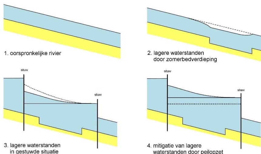
Figuur 2.19: Schematische weergave van de werking van zomerbedverdiepingen.
