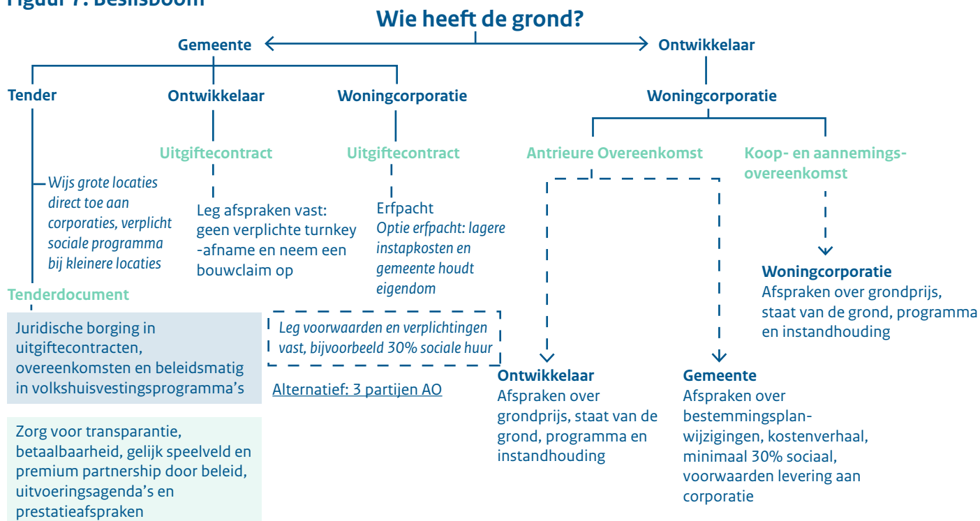
Figuur 7: Beslisboom
