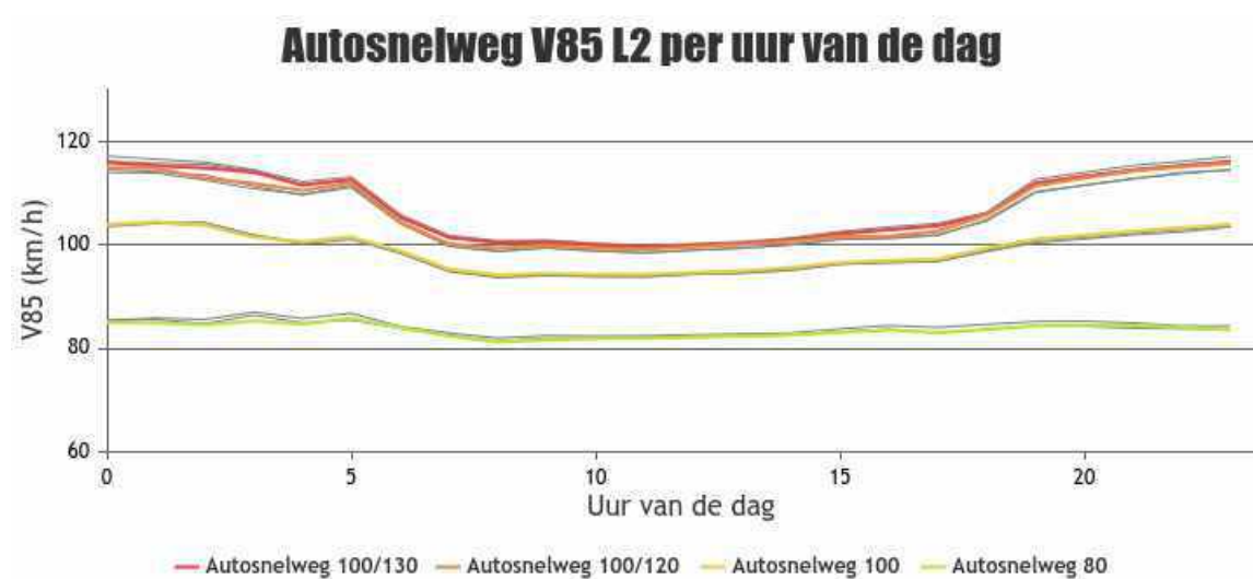
Afbeelding 9.4 De V85 per uur van de dag op autosnelwegen voor L2; 2024 is met gekleurde lijnen ingetekend voor de verschillende regimes, 2022 en 2023 zijn grijs ingetekend ter referentie
