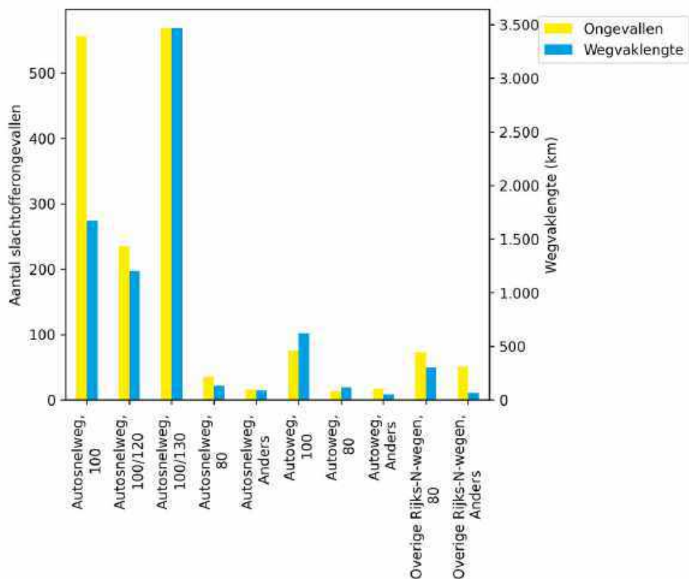
Afbeelding 3.10 Aantal slachtofferongevallen en wegvaklengte naar wegtype en snelheidslimiet 2022-2024 (bron: BRON, NWB, WEGGEG, INWEVA)
