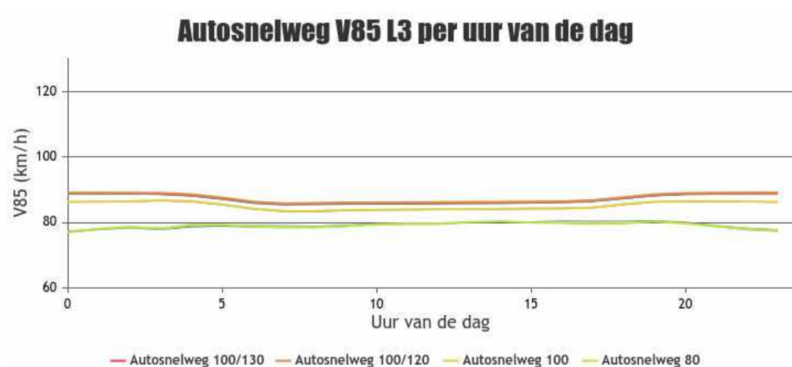
Afbeelding 9.5 De V85 per uur van de dag op autosnelwegen voor L3; 2024 is met gekleurde lijnen ingetekend voor de verschillende regimes, 2022 en 2023 zijn grijs ingetekend ter referentie
