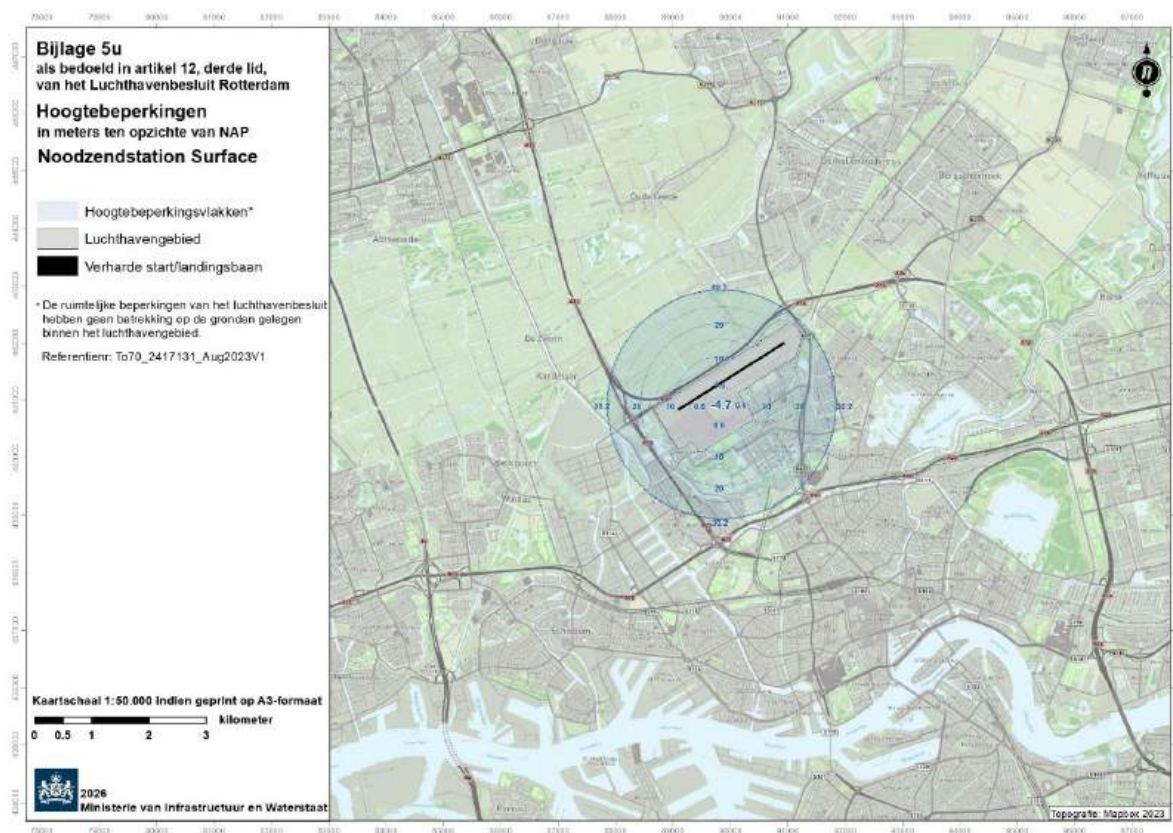
Bijlage 5u als bedoeld in artikel 12, derde lid, van het Luchthavenbesluit Rotterdam Kaart (1:50.000) met hoogtebeperkingen: Surface voor noodzendstation
