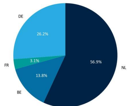
Binnenvaart transportprestatie in Rijnvaartlanden excl. CH D08: Bouwmaterialen in 2023
