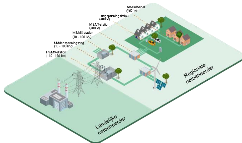
Figuur 2: Regelstation en schakelstation in perspectief van het grotere energienetwerk. Bron: Witteveen+Bos
