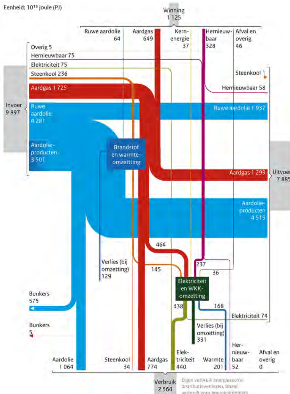
Figuur 9.8: Energiestromen in PJ (CBS, 2022)
