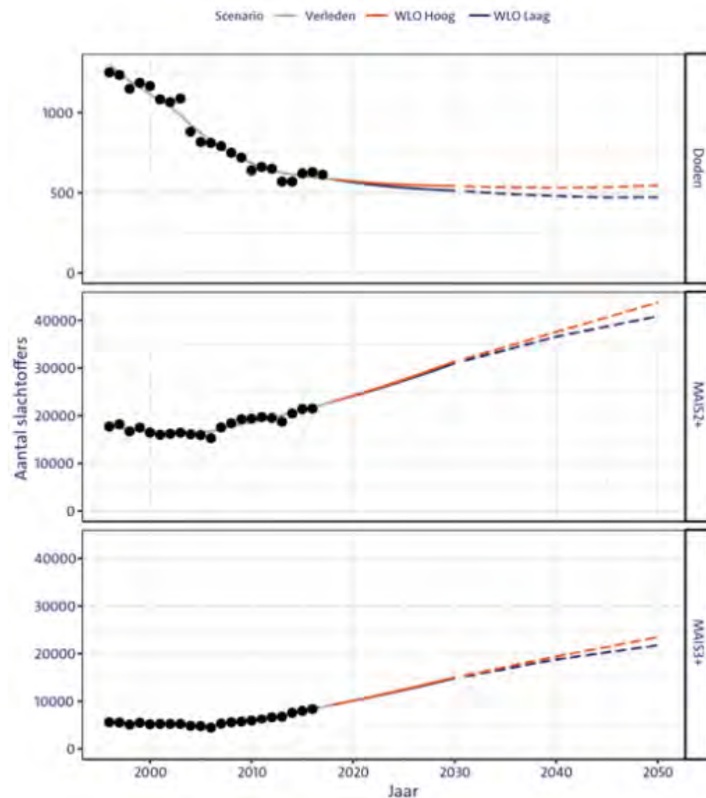
Figuur 2.14: Prognose verkeersslachtoffers: doden, MAIS2+, MAIS3+ (Bron: SWOV, 2022) 5
