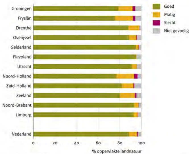
Figuur 5.22: Geschiktheid van milieuconditie zuurgraad voor landnatuur per provincie (Bron: CLO, 2020)
