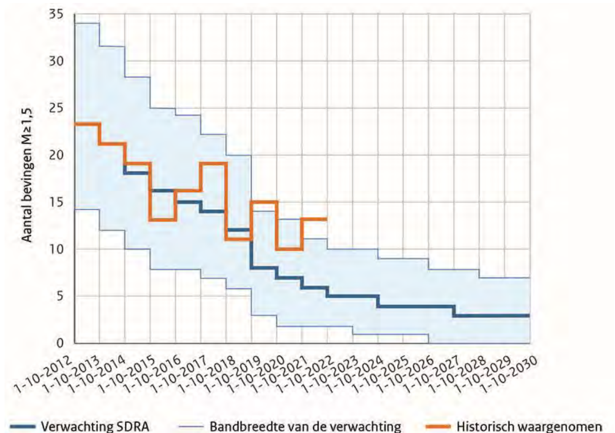
Figuur 2.11: Overzicht van het aantal waargenomen bevingen per gasjaar (oranje) en de verwachting op basis van de SDRA-berekening uit 2021 (blauw) (Bron: Staatstoezicht op de Mijnen, n.d.)
