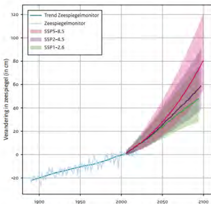
Figuur 2.7: Zeespiegel zoals waargenomen aan de Nederlandse kust en volgens de indicatieve zeespiegelprojecties (Bron: KNMI, 2021)
