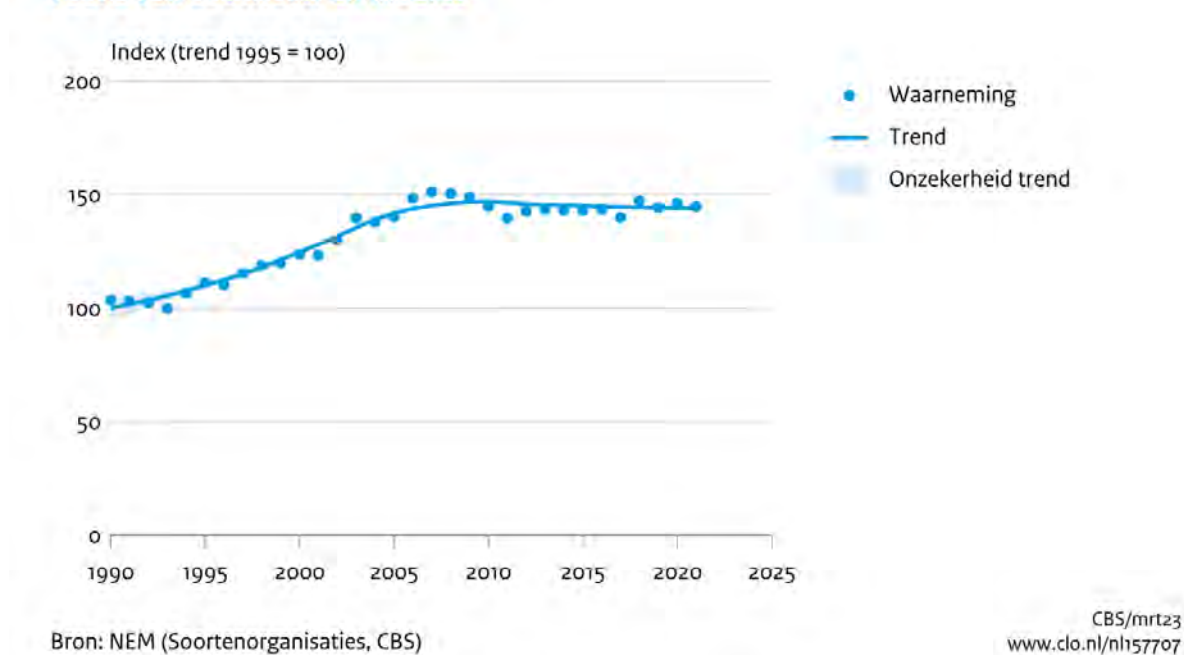
Figuur 5.9: Fauna van zoetwater en moeras (CLO, 2023)
