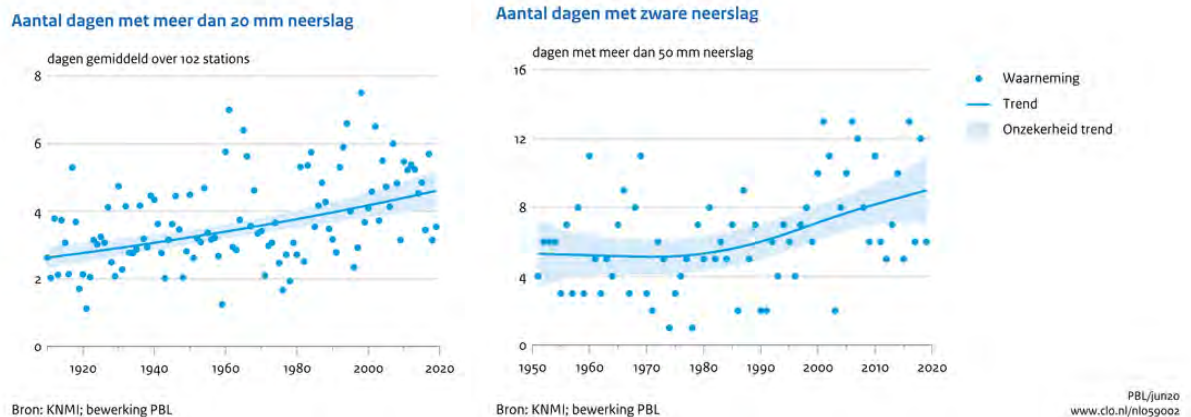
Figuur 3.13: Trend aantal dagen met meer dan 20 mm neerslag (links) en meer dan 50 mm neerslag (rechts) (CLO, 2020)
