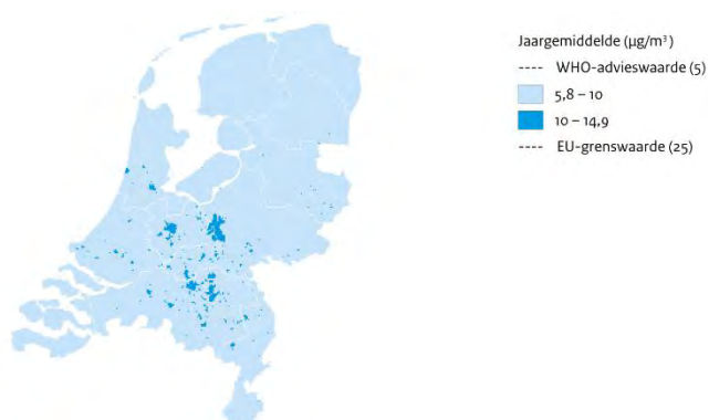
Figuur 1.6 Concentraties zeer fijn stof ( \text{PM}_{2.5} ) in 2022 (RIVM, 2023)
