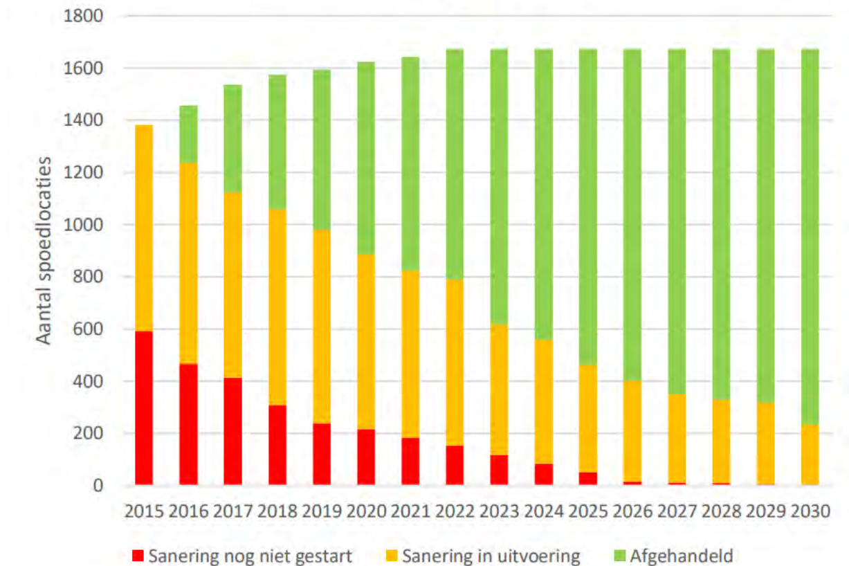
Figuur 4.11: Voortgang aanpak bodemverontreiniging (Bron: Ministerie van Infrastructuur en Waterstaat, 2022)
