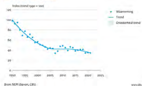
Figuur 5.11: Fauna van bos (Bron: CLO, 2023) en Fauna in open natuurgebieden (Bron: CLO, 2023)
