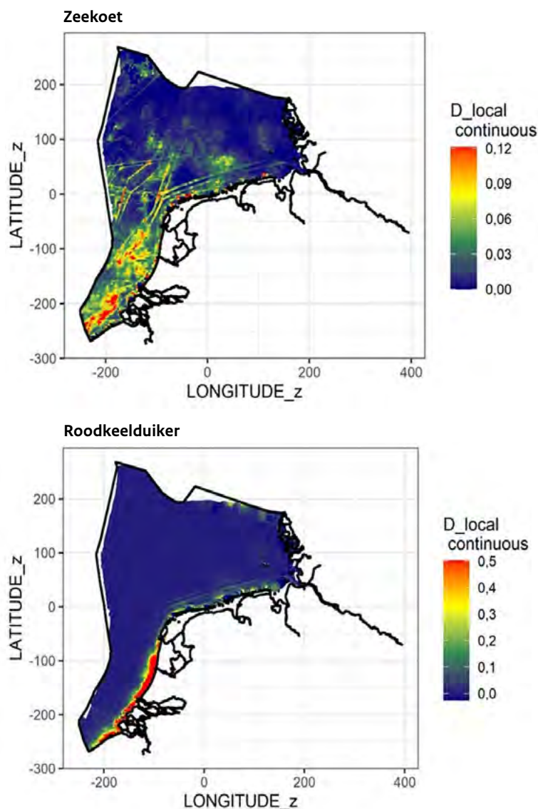
Figuur 1.1.4. Ruimtelijke verdeling in de Duitse, Nederlandse en Belgische delen van de Noordzee van D_{\text{local}} , de maat voor verstoring door menselijke activiteiten in de OSPAR pilot indicator B7, voor zeekoet (boven) en roodkeelduiker (onder). Een hoge D_{\text{local}} geeft aan dat op die plek veel minder vogels aanwezig zijn dan in een modelscenario zonder verstoringbronnen. De verspreiding van beide soorten wordt negatief beïnvloed door scheepvaart en windparken op zee. Duidelijk is de samenhang te zien tussen zones met het grootste verstoringseffect en het natuurlijke leefgebied van zeevogels: de roodkeelduiker is veel meer kustgebonden dan de zeekoet. Een optelling van de D_{\text{local}} -waarden, gewogen naar de lokale onverstoorte vogeldichtheid, geeft een verstoringmaat voor het gehele verspreidingsgebied van de soort. Voor zeekoet en roodkeelduiker bedraagt D_{\text{global}} respectievelijk 0.10 en 0.41, wat betekent dat volgens de schattingen uit het statistische model in de huidige situatie 10 procent en 41 procent minder individuen in het studiegebied aanwezig zijn dan in een situatie zonder verstoringbronnen (uit Dierschke & Mercker 2022).
