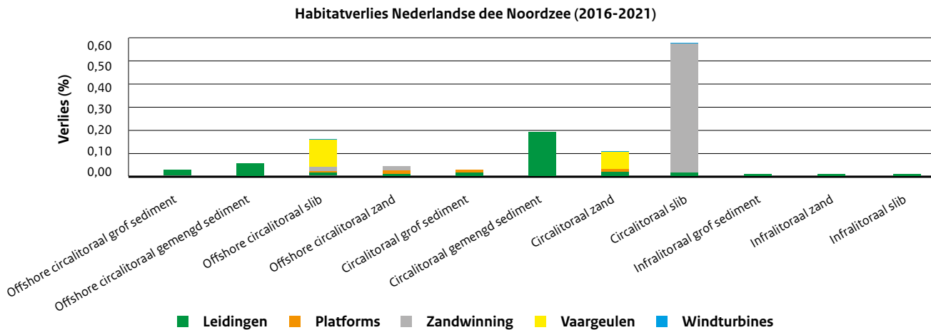
Figuur 6.9. Habitatverlies (%) in het Nederlandse deel van de Noordzee over de periode 2016-2021 per breed habitattypen (BHT), waarbij de bijdragen van verschillende structuren/activiteiten inzichtelijk zijn gemaakt. Verlies door visserij is geen onderdeel van de Nederlandse analyse en is hier daarom buiten beschouwing gelaten. Volgens OSPAR bedraagt dit verlies 1,5% van het offshore circalitoraal slib.
