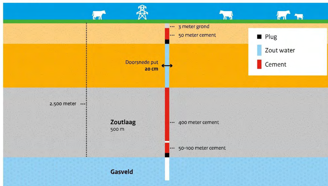
Figuur 5.1.3.1 Schematische tekening van putafsluiting in het Groningen-gasveld
