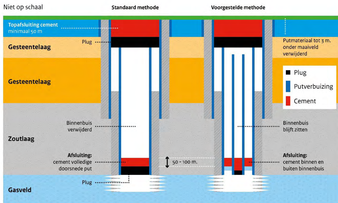
Figuur 5.1.3.2 Overzicht van de tubing in een werkende put, bij standaard afsluiting en bij TTA-afsluiting
