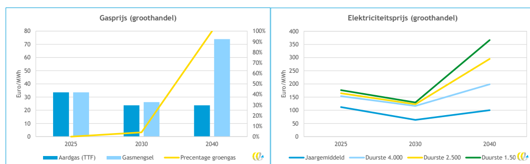
Figuur 3 - Aangenomen groothandelsprijzen voor gas (inclusief bijmenging) en elektriciteit
