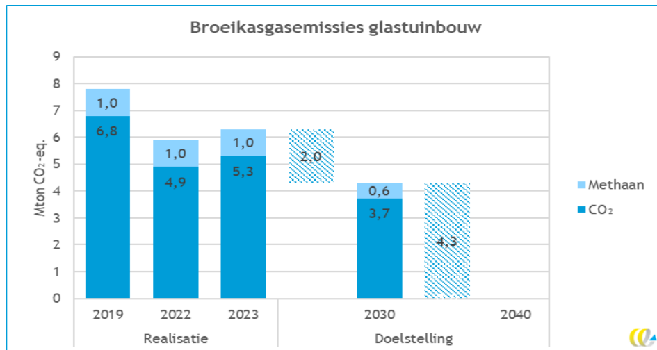
Figuur 2 - Gerealiseerde emissies, emissiedoelstellingen en benodigde emissiereductie in de glastuinbouw
