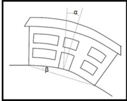
Figuur 15.: Skew ( \alpha ) en relatieve kromming ( \beta ).
