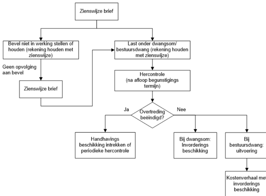
Schema reactie 1
