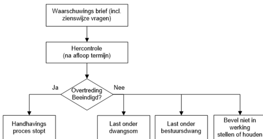
Schema reactie 2
