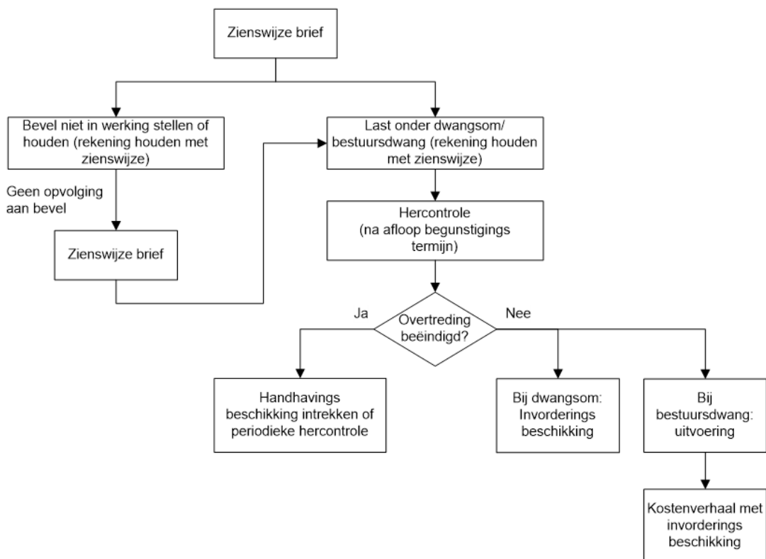
Schema reactie 1
