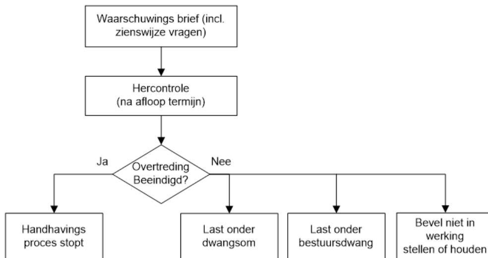
Schema reactie 2
