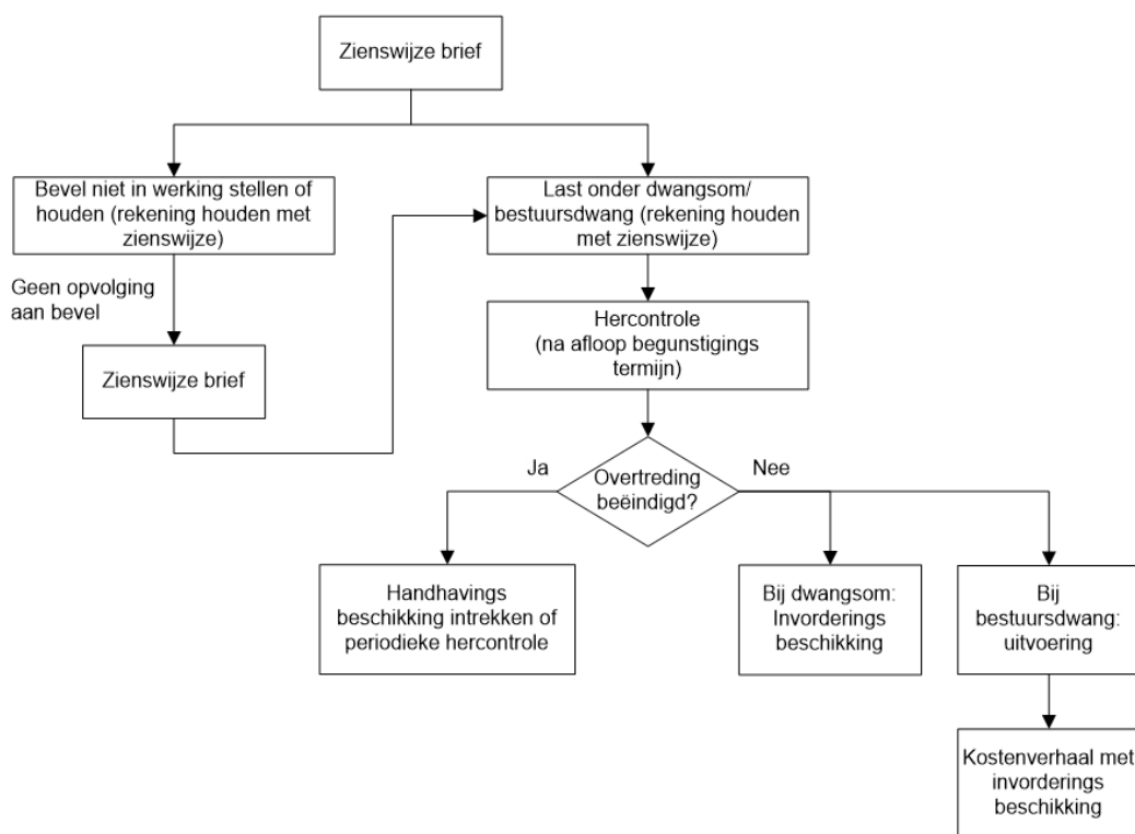
Schema reactie 1
